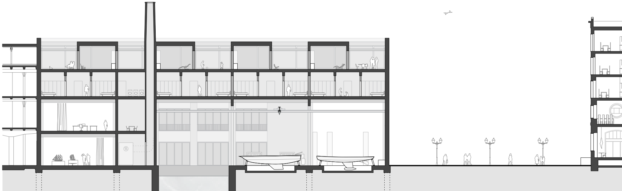
Längsschnitt A_A
