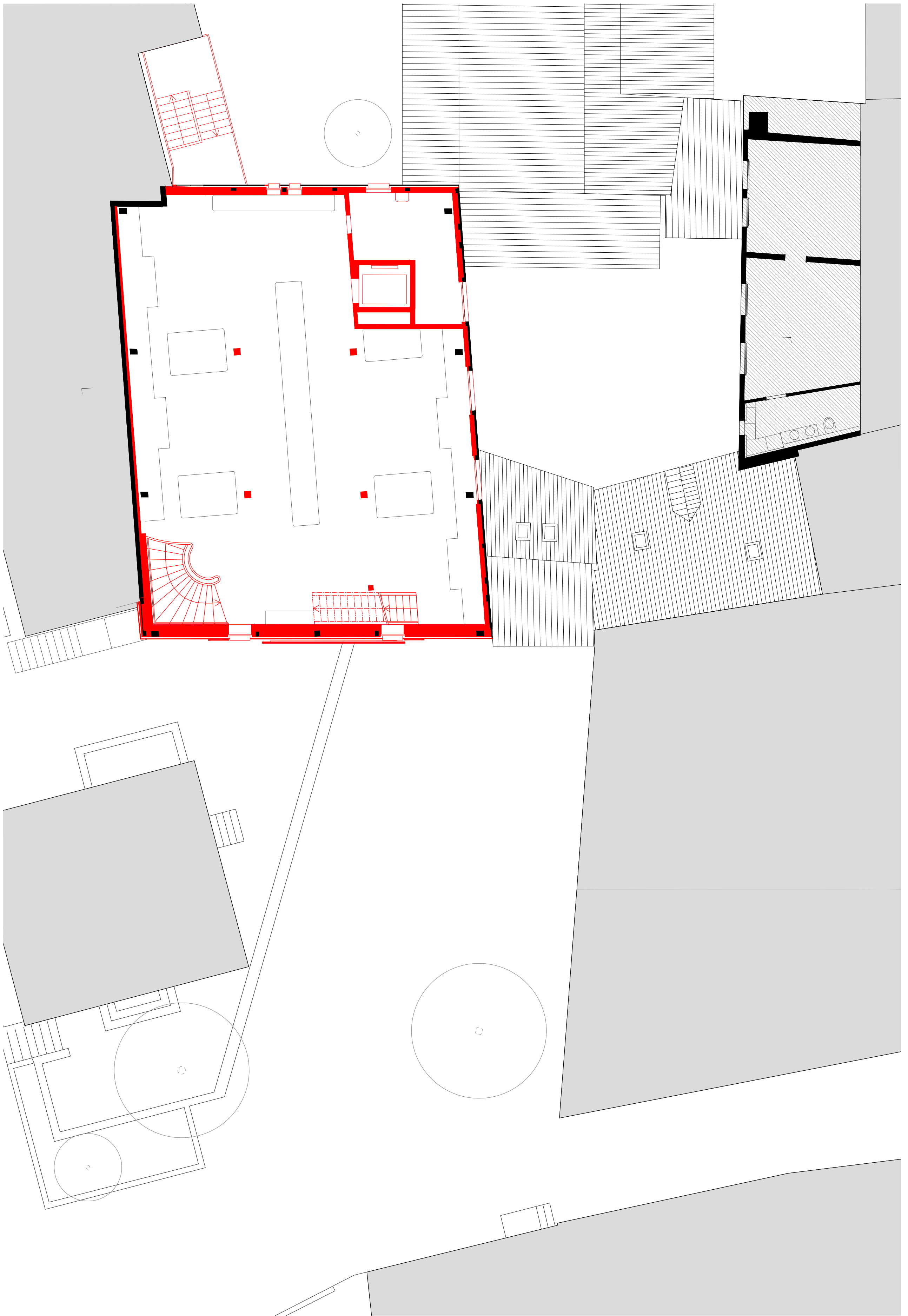
2. Obergeschoss
