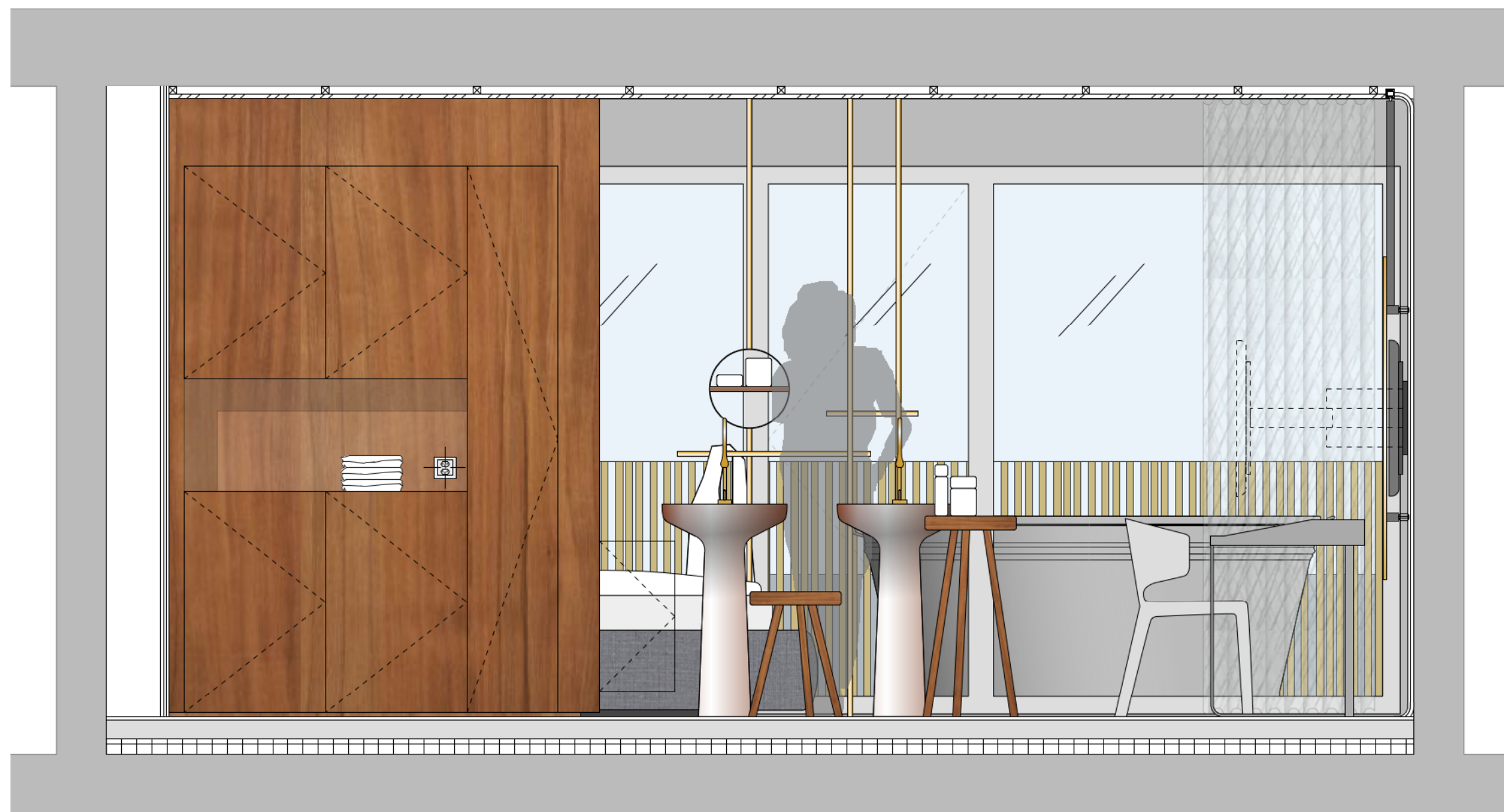
Querschnitt | Mst. 1:20
