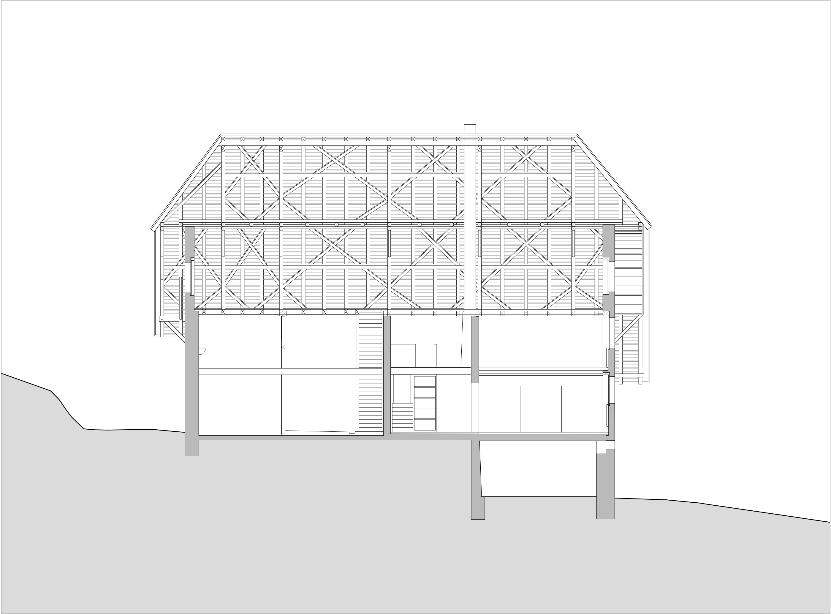
langschnitt/coupe longitudinale B
