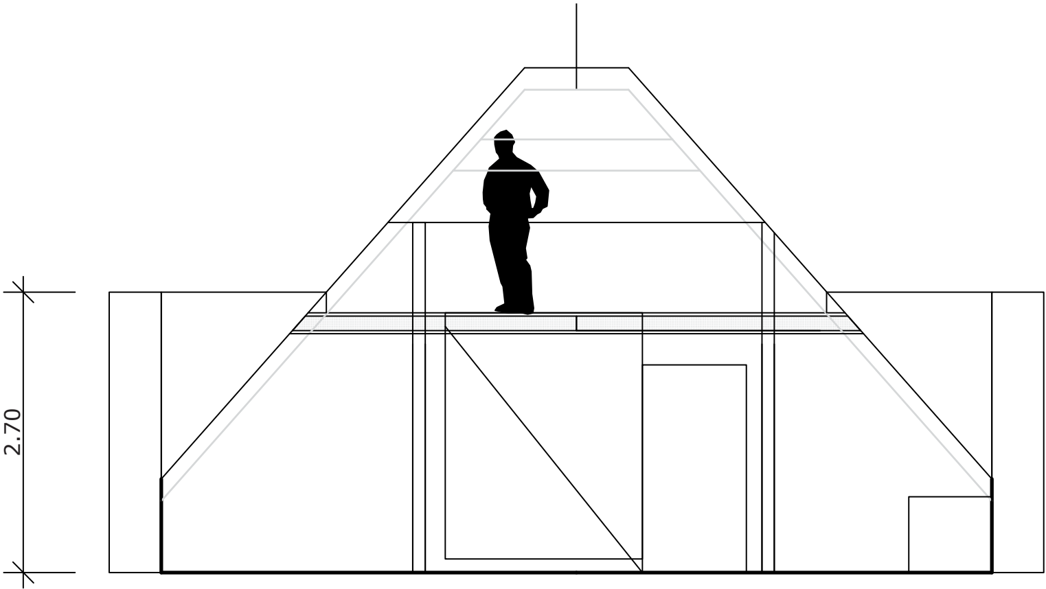
Längsschnitt
