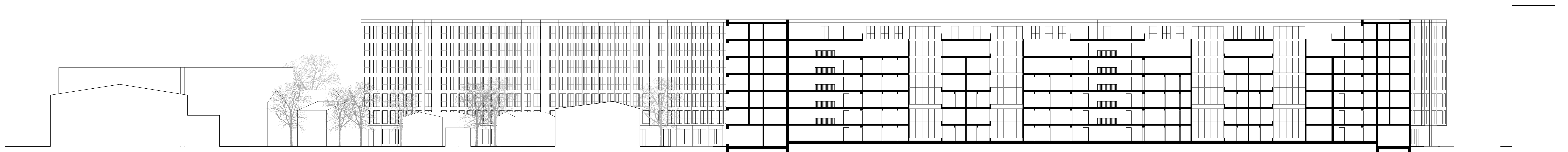
Schnitt C 1:250
