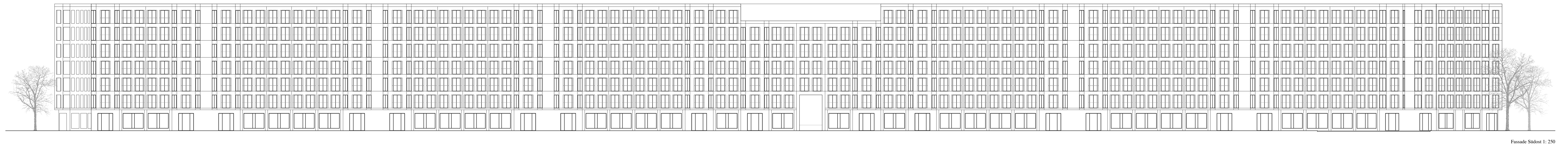
Fassade Südost 1:250
