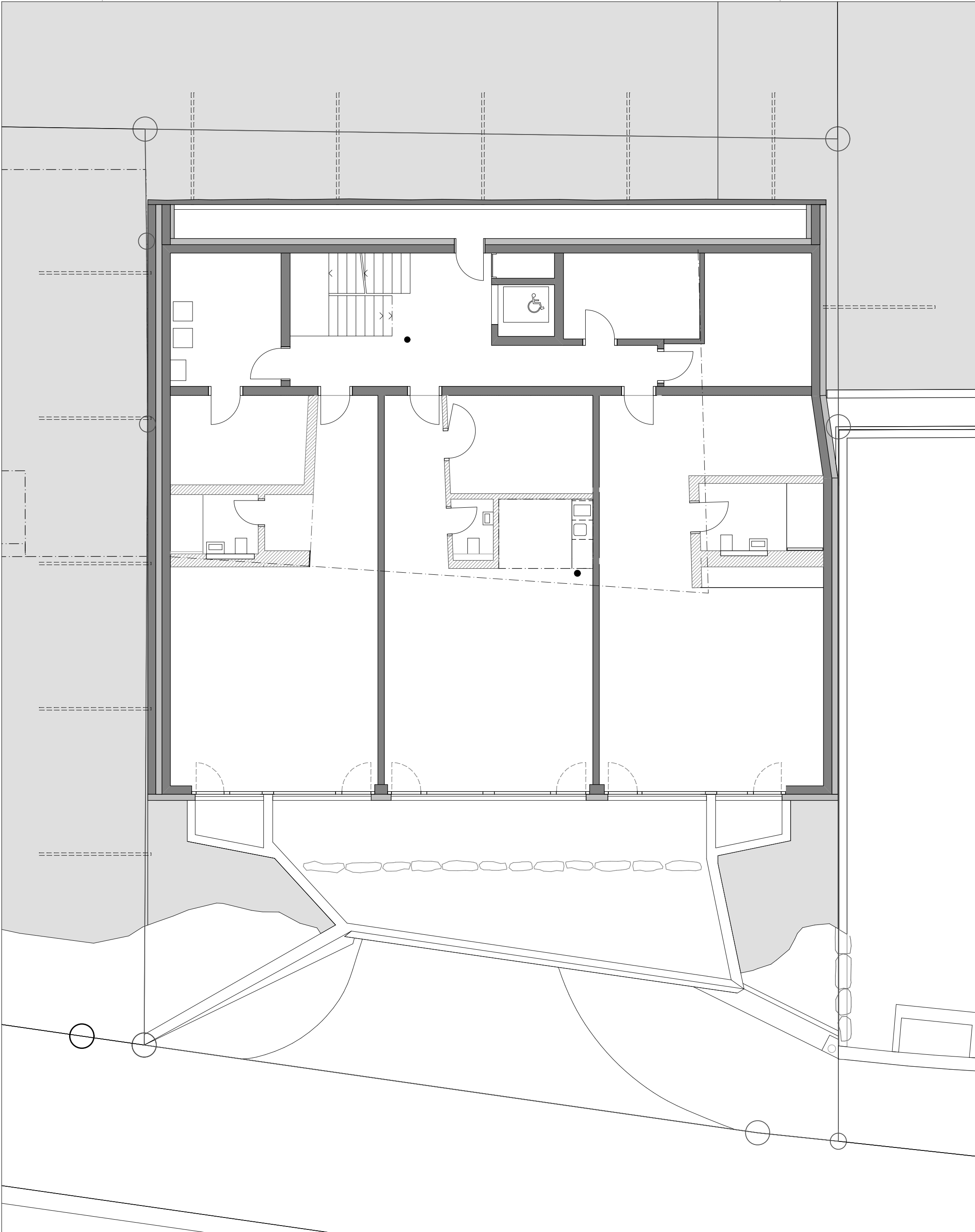
GRUNDRISS ERDGESCHOSS
