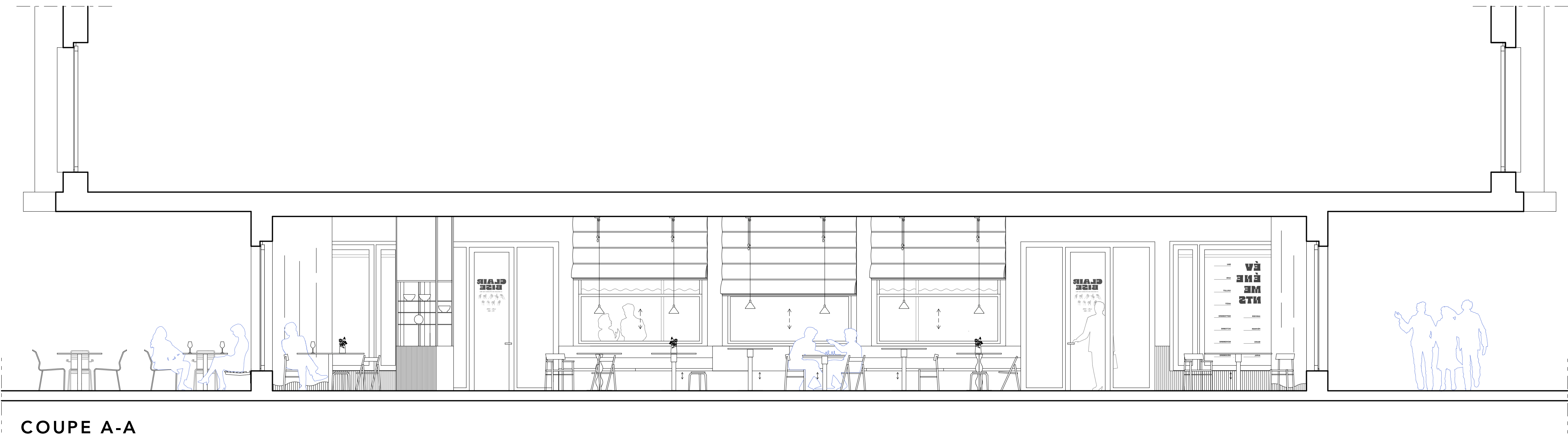
COUPE A-A
