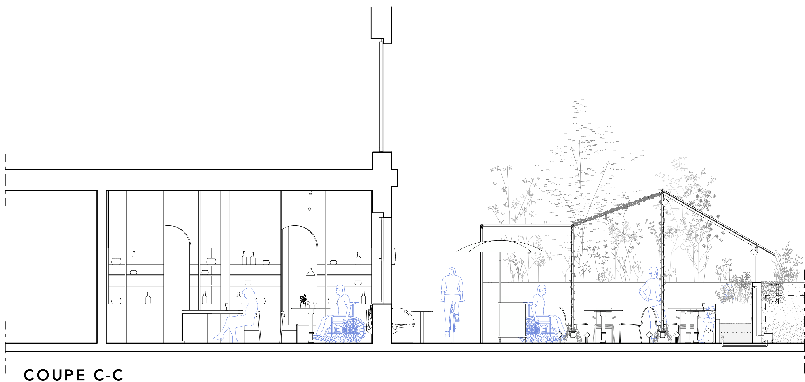
COUPE C-C
