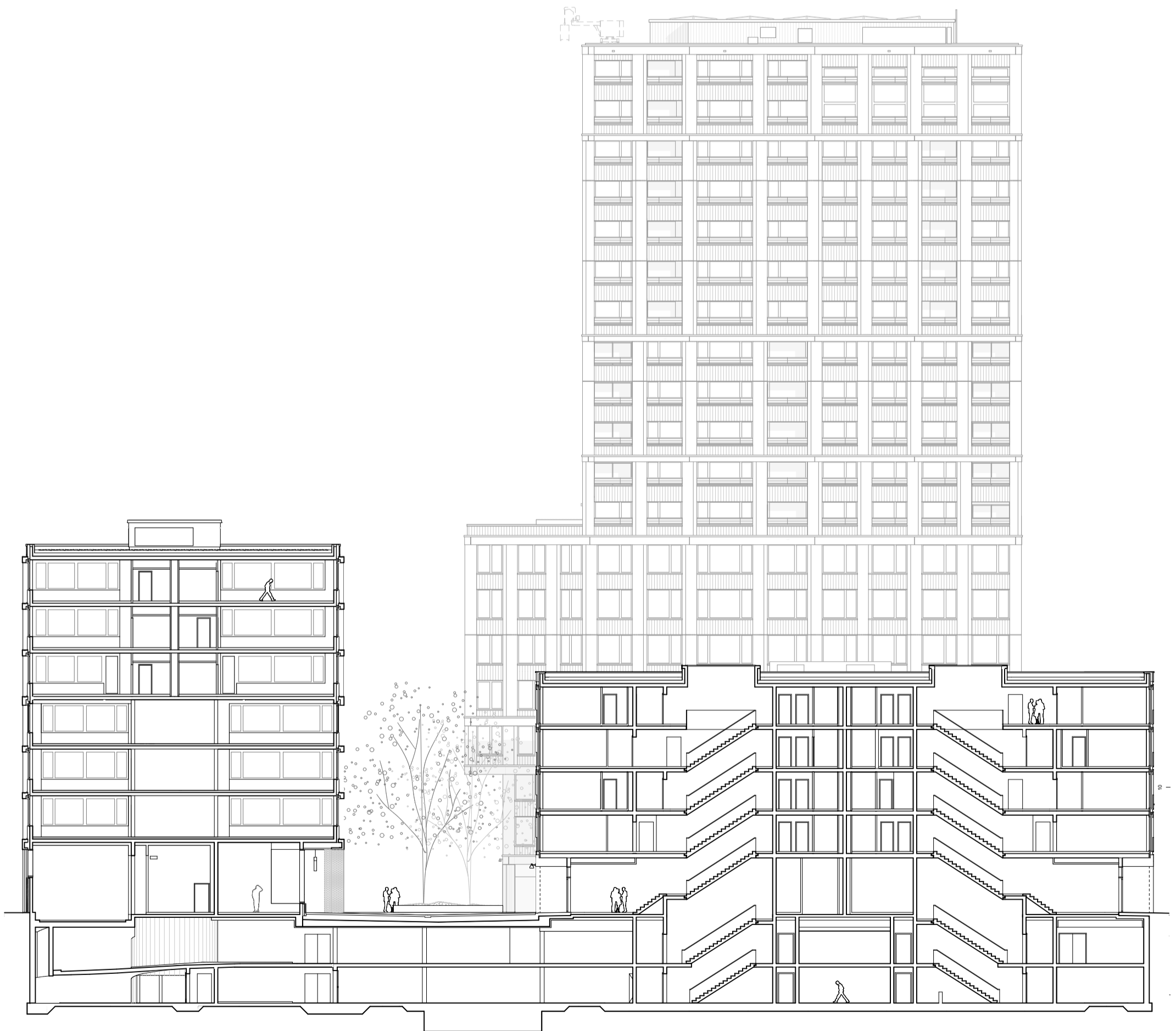
Coupes et élévations sur façades sud
