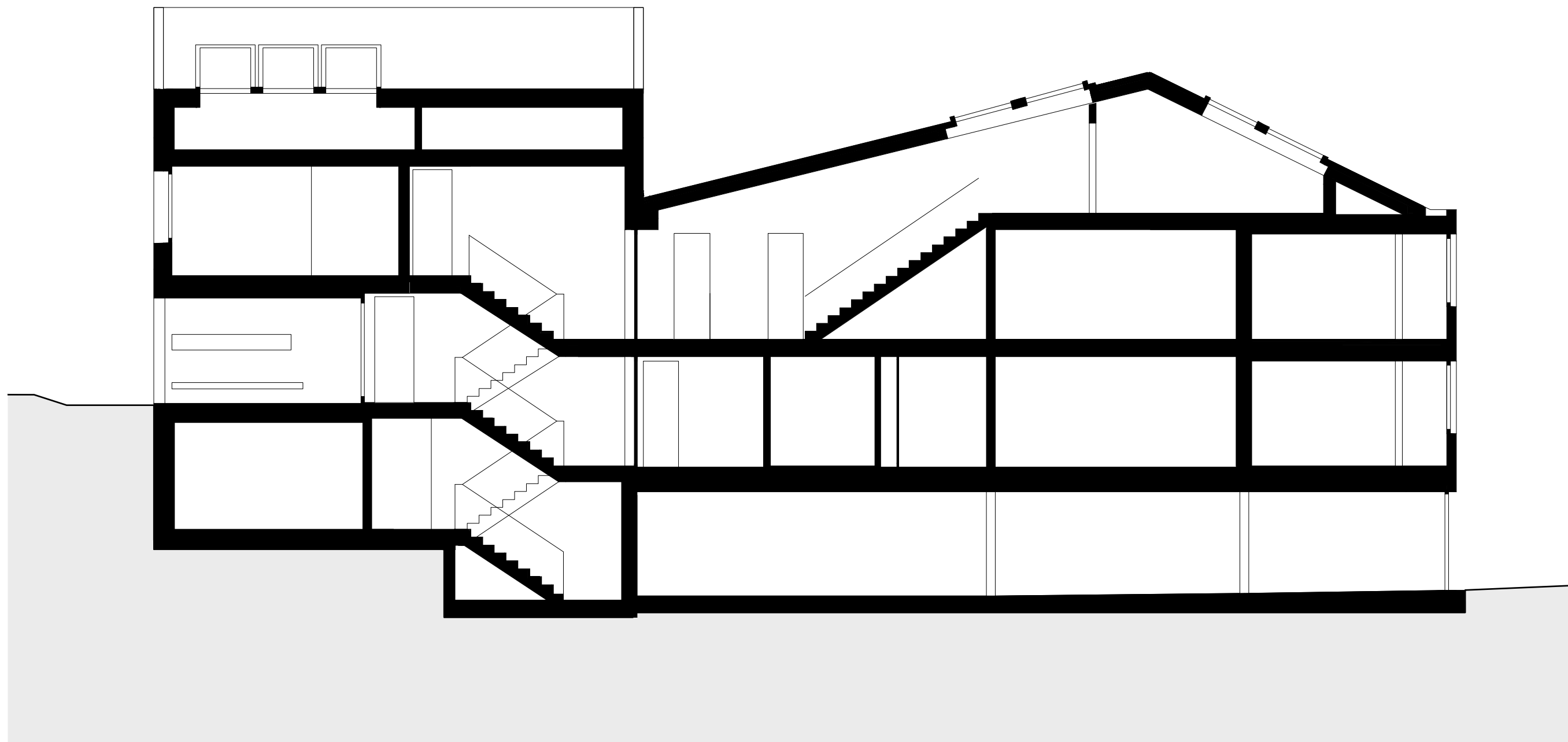
Längsschnitt 1:100
