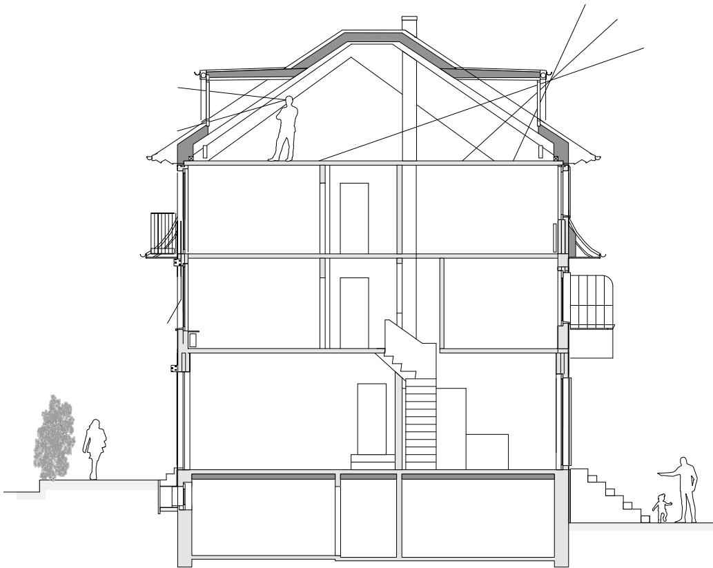
Schnitt A-A Haus Nr. 7a
