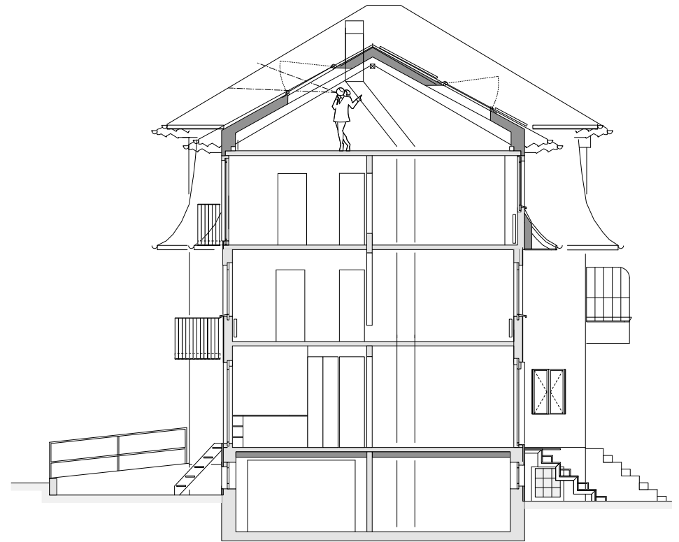
Schnitt B-B Haus Nr. 9
