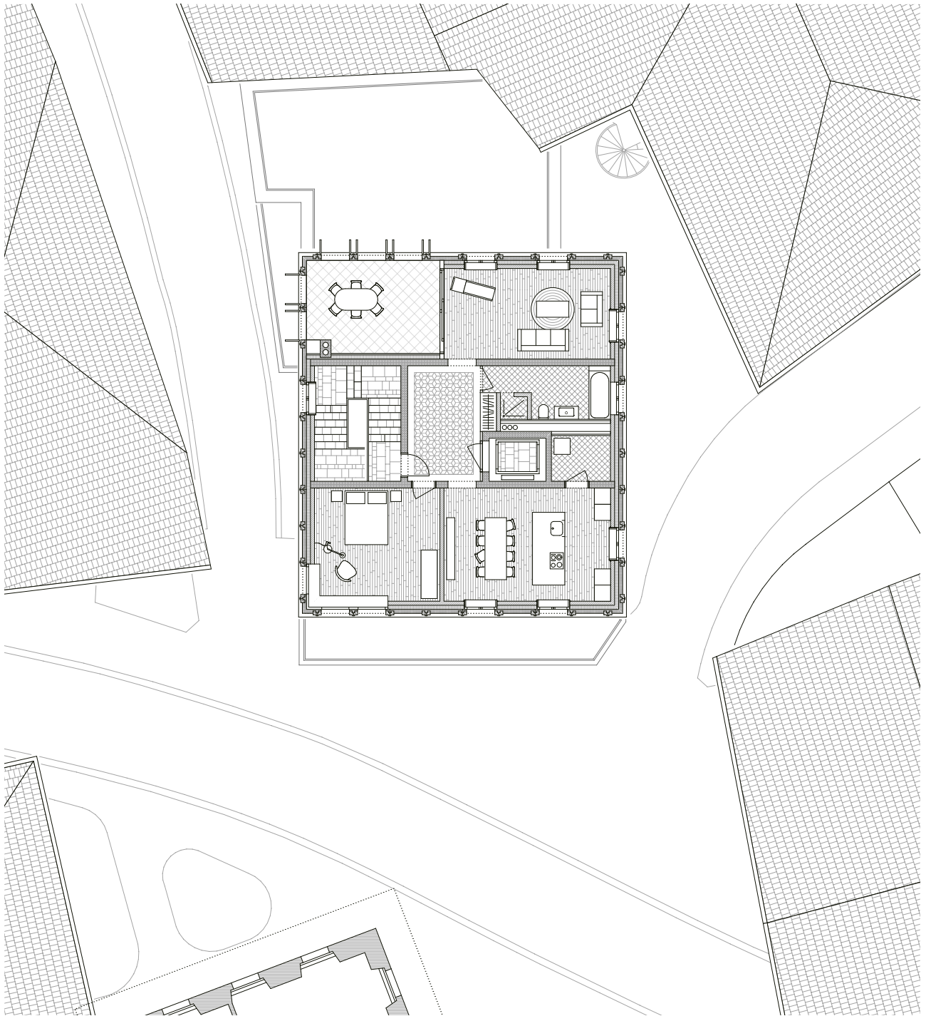
DACHGESCHOSS 1:200 ☉
