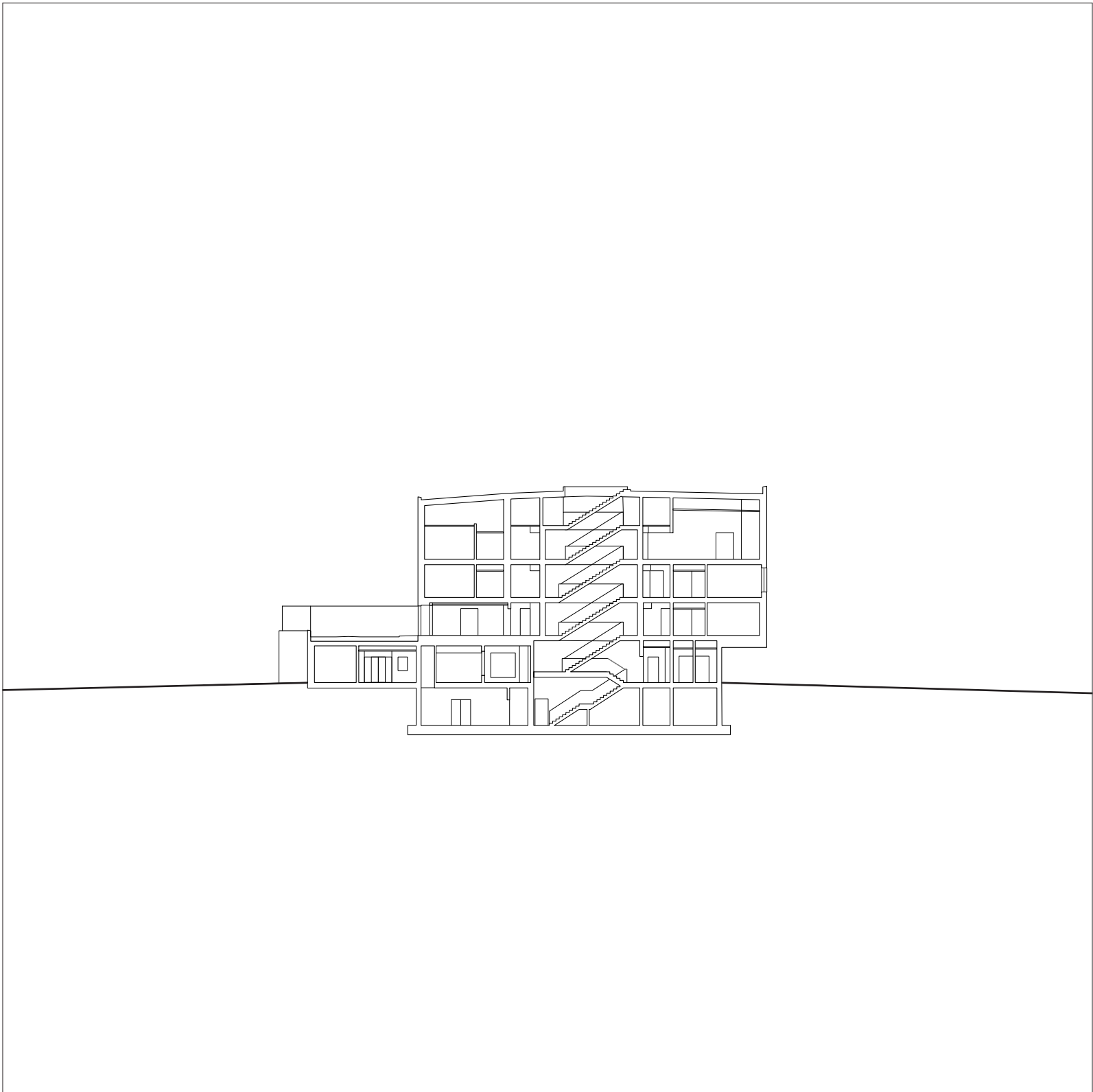
COUPE TRANSVERSALE 0 15
