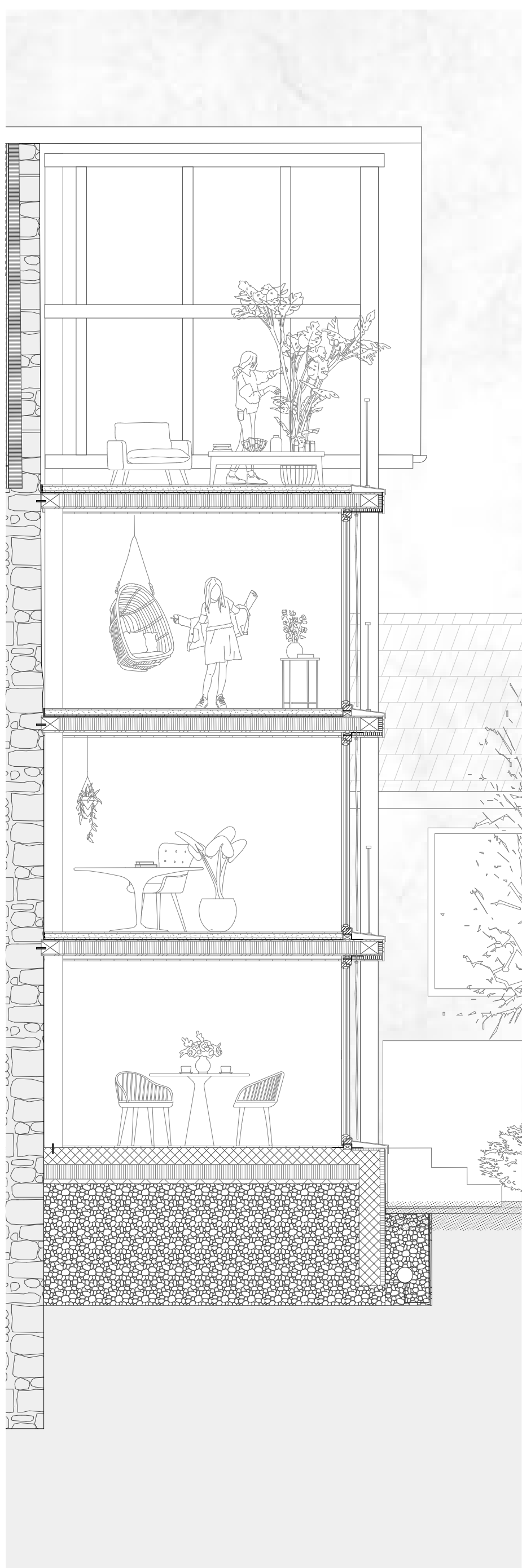
Fassadenschnitt 1:50
