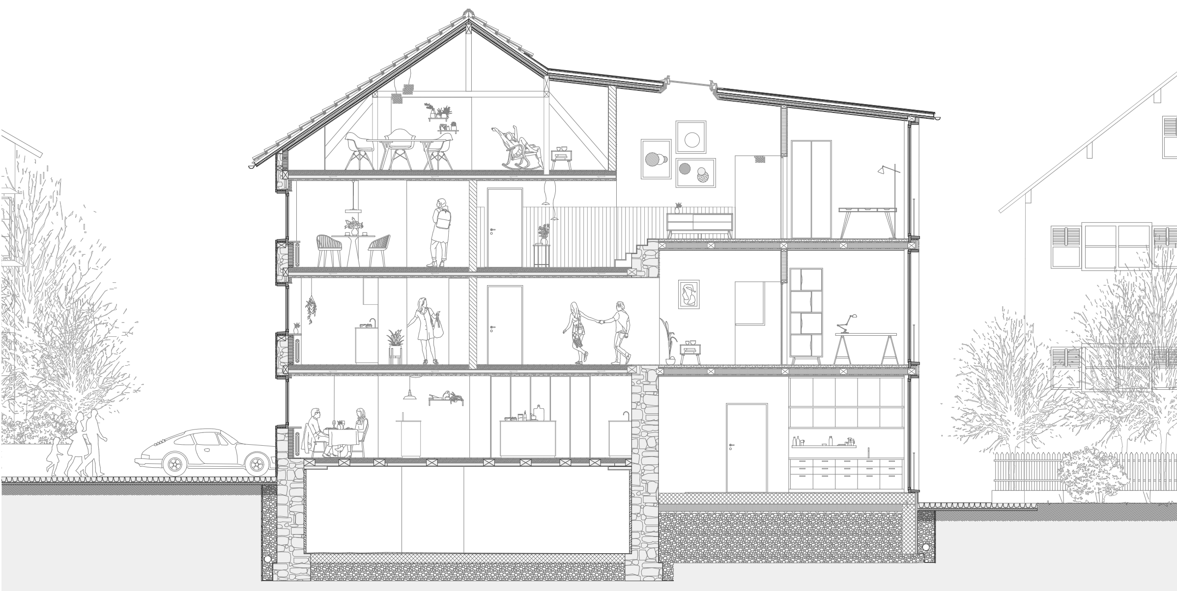
Schnitt 1:100
