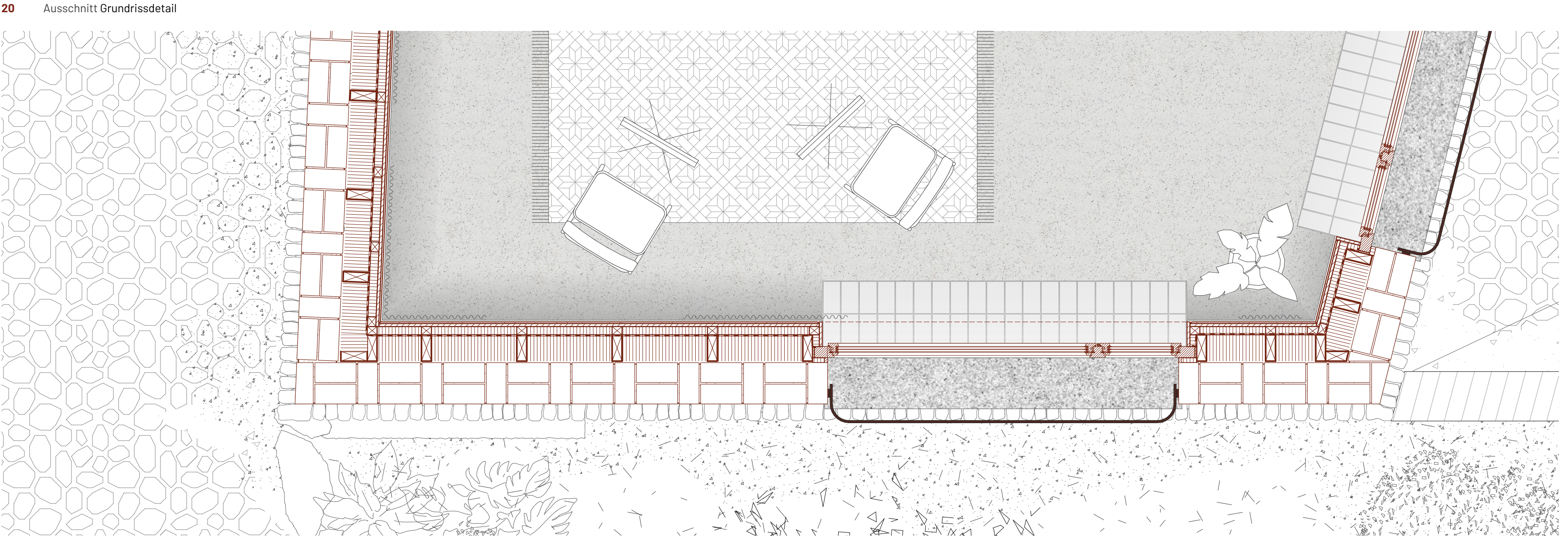
20 Ausschnitt Grundrissdetail
