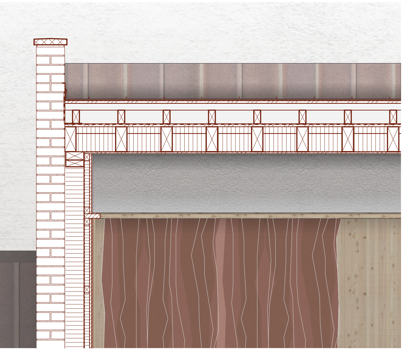
20 Ausschnitt Anschluss Dach
