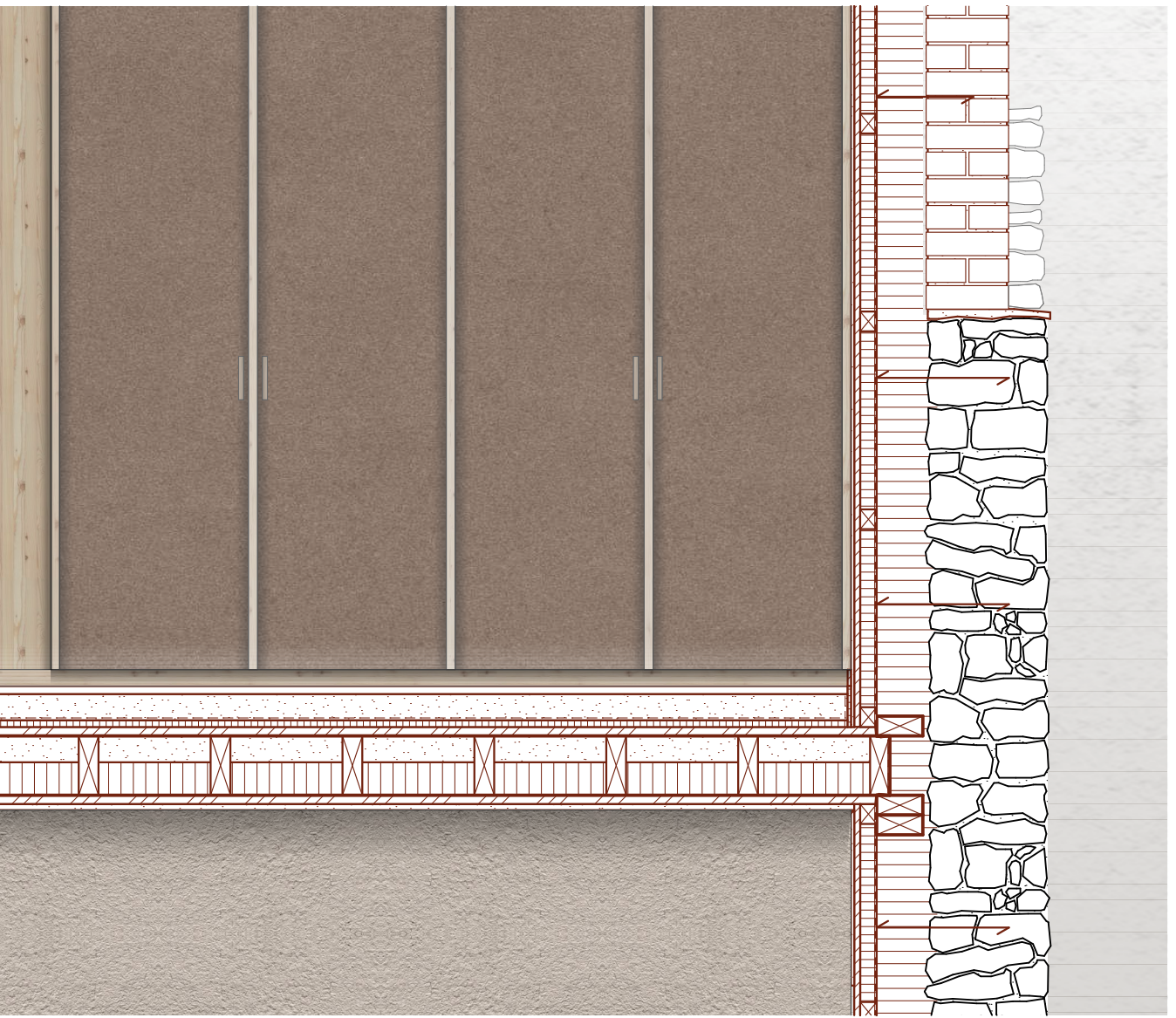
20 Ausschnitt Anschluss Wand
