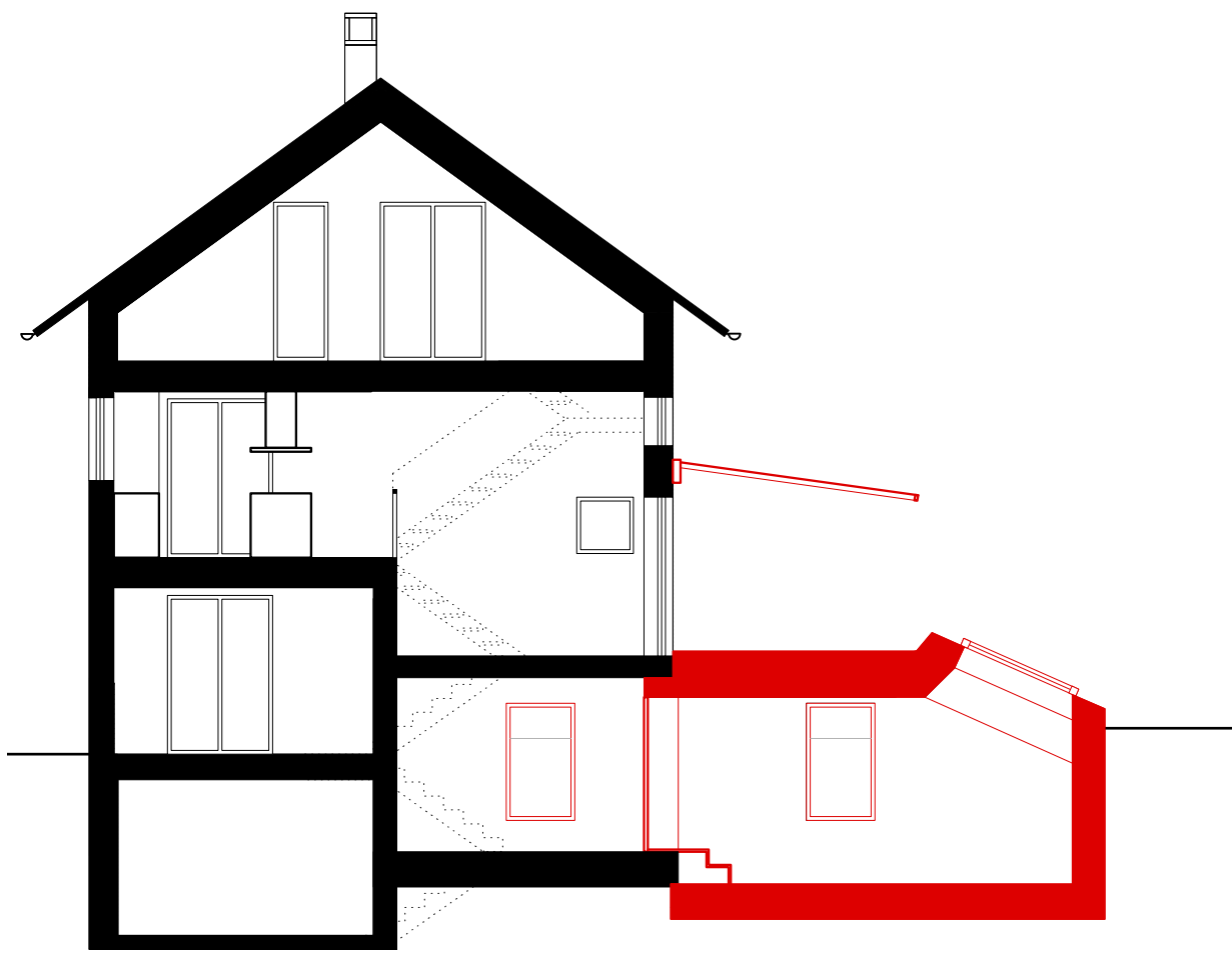
Querschnitt
