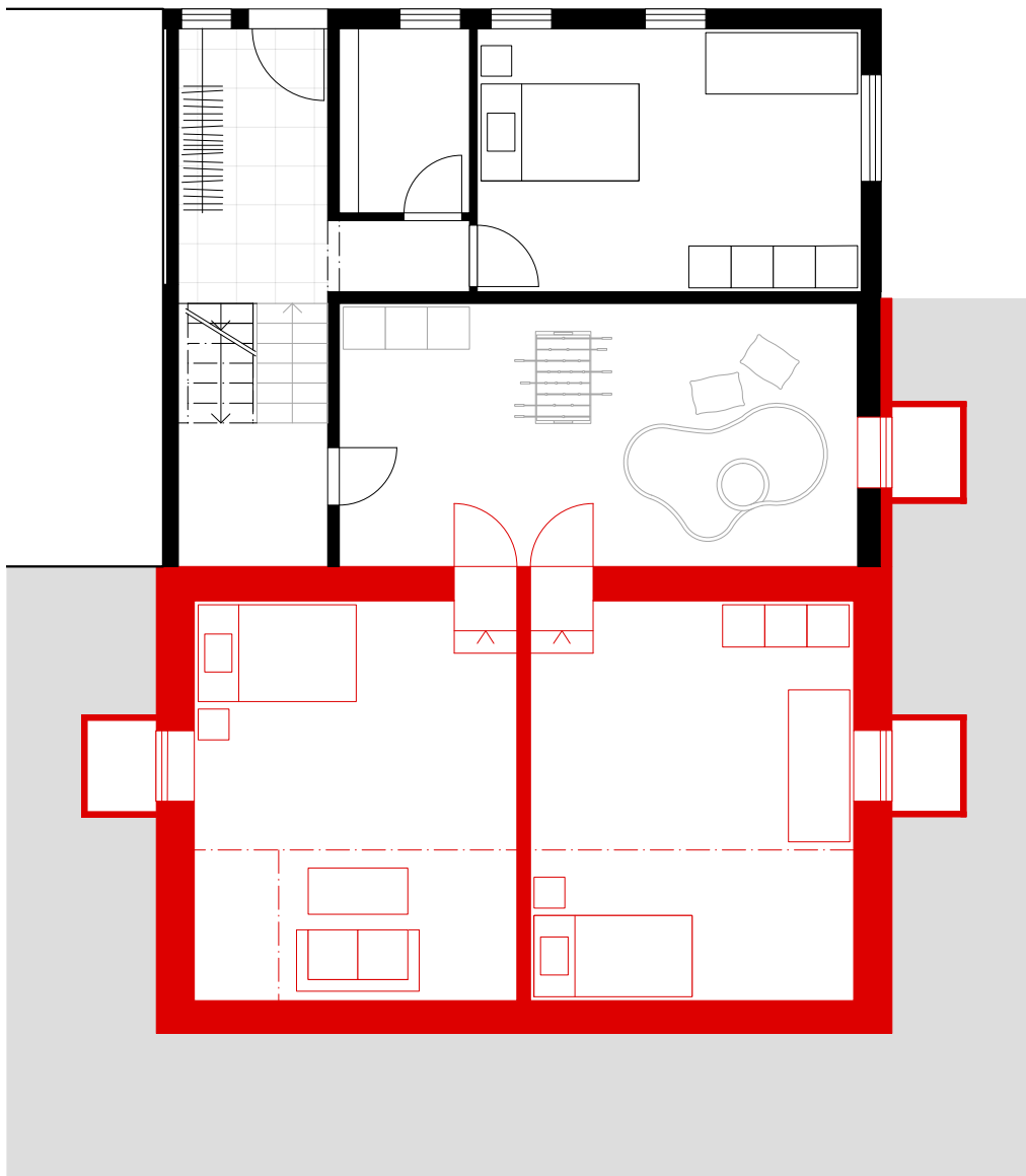
Grundriss Zimmer
