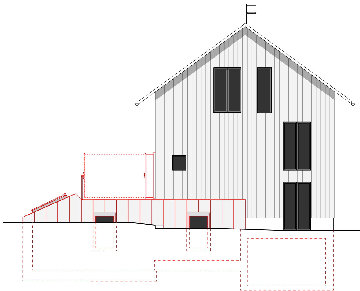
Ansicht Ost
