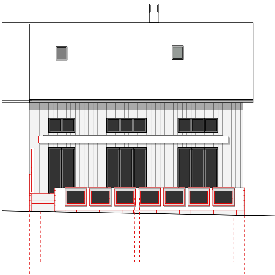
Ansicht Süd
