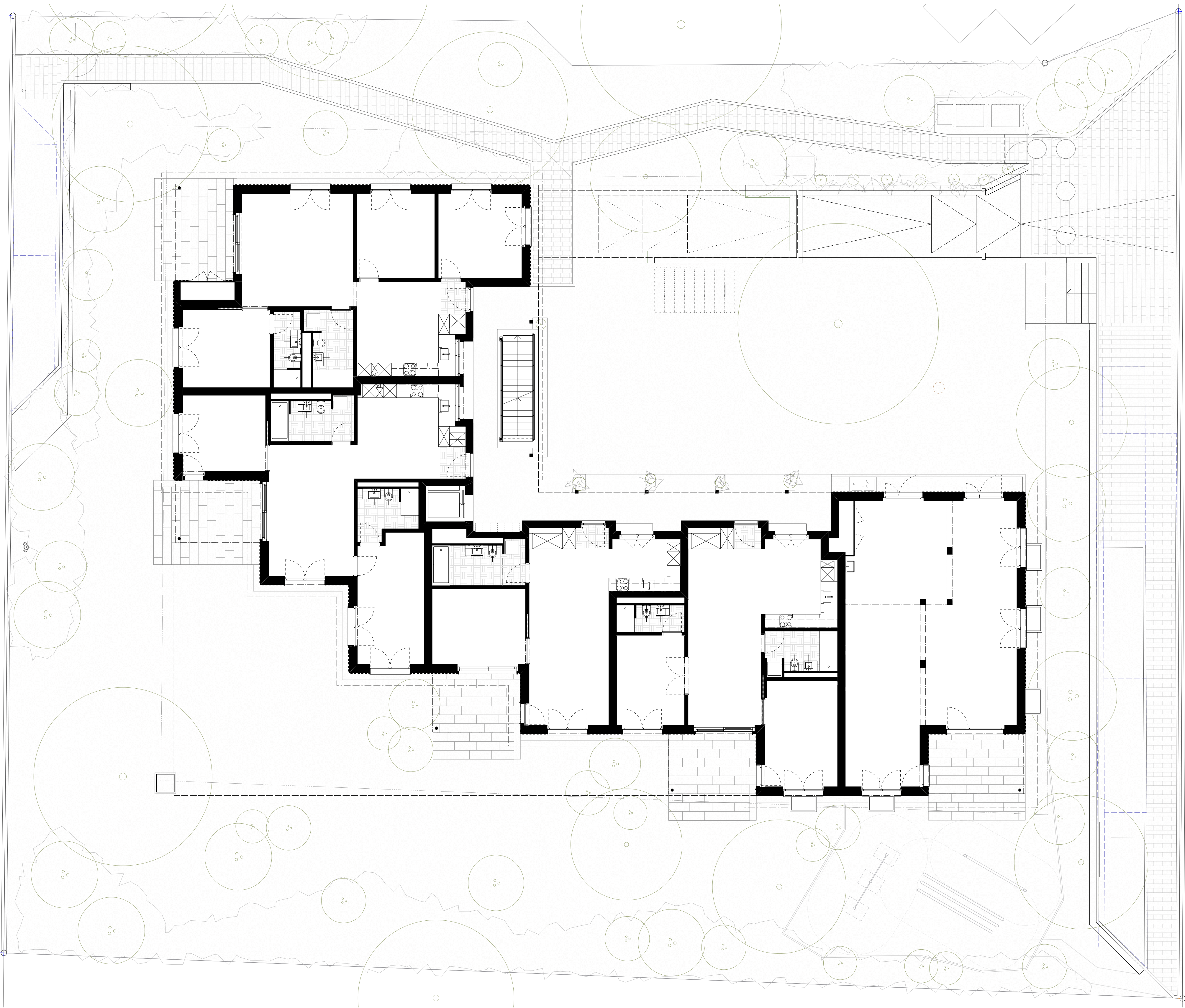
Zum Grünen Hof - Fehrltorf Grundriss Erdgeschoss
