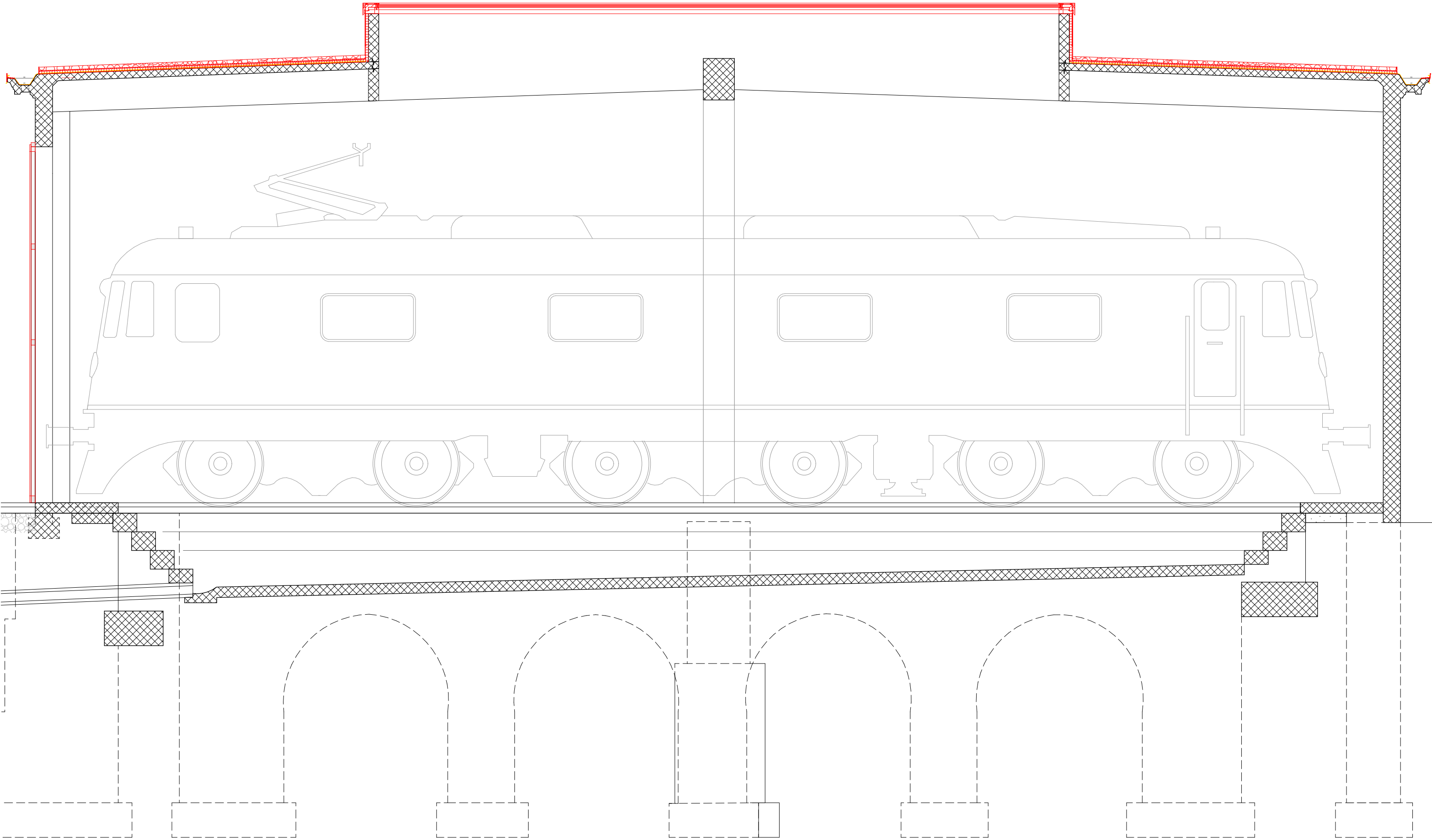
Querschnitt 1:50
