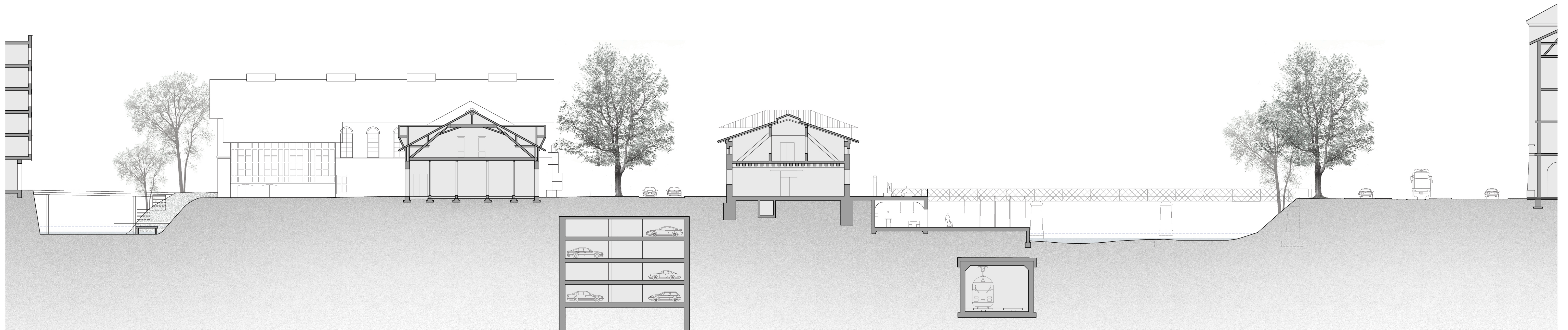
Schnitt a-a
