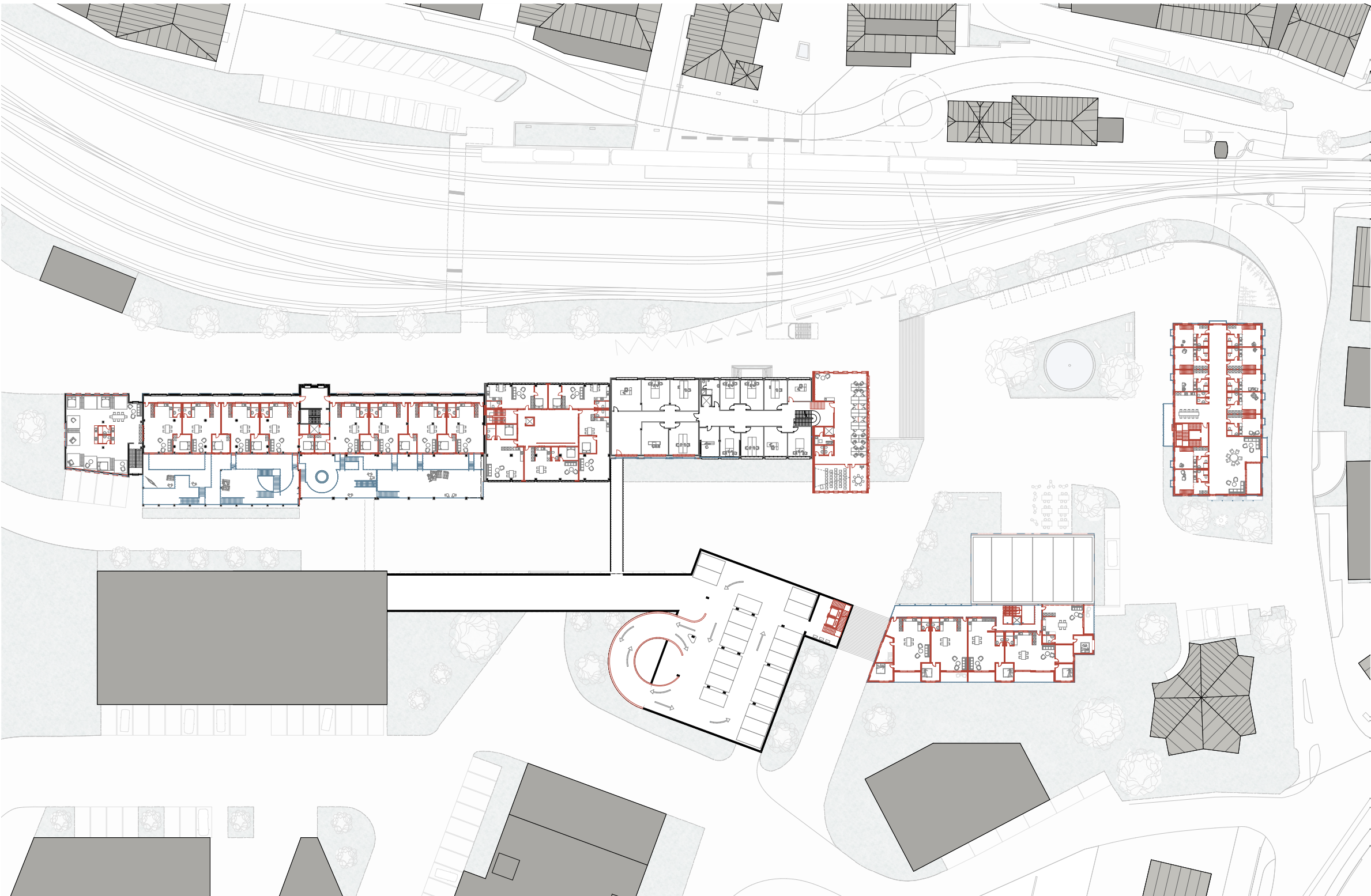
Regelgrundriss, Niveau +1
