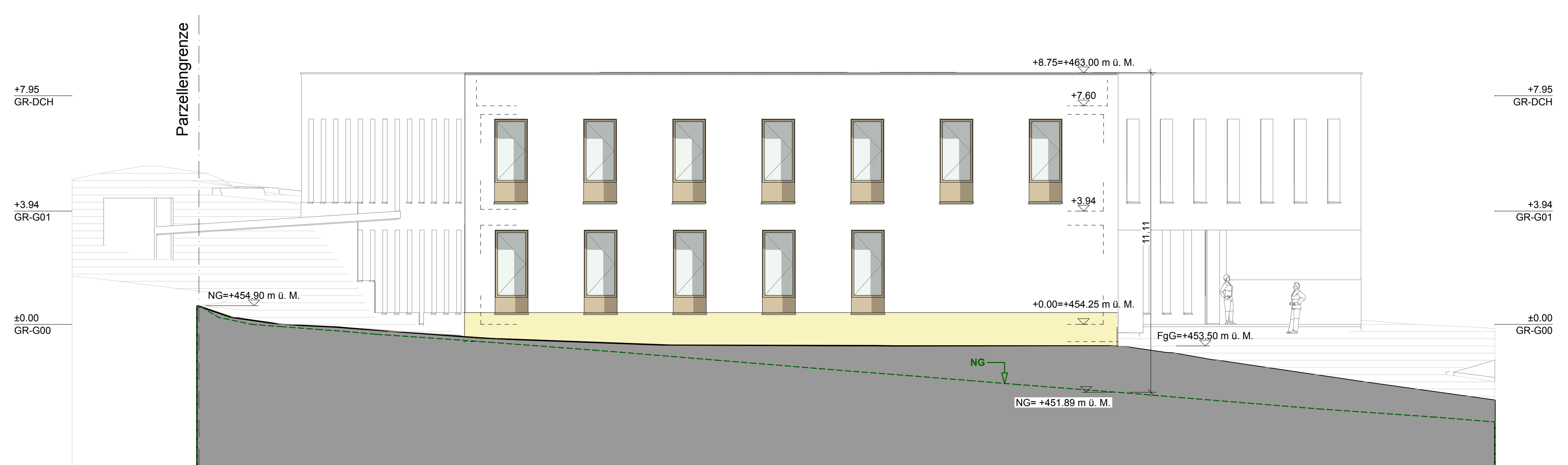
Ansicht Nord
