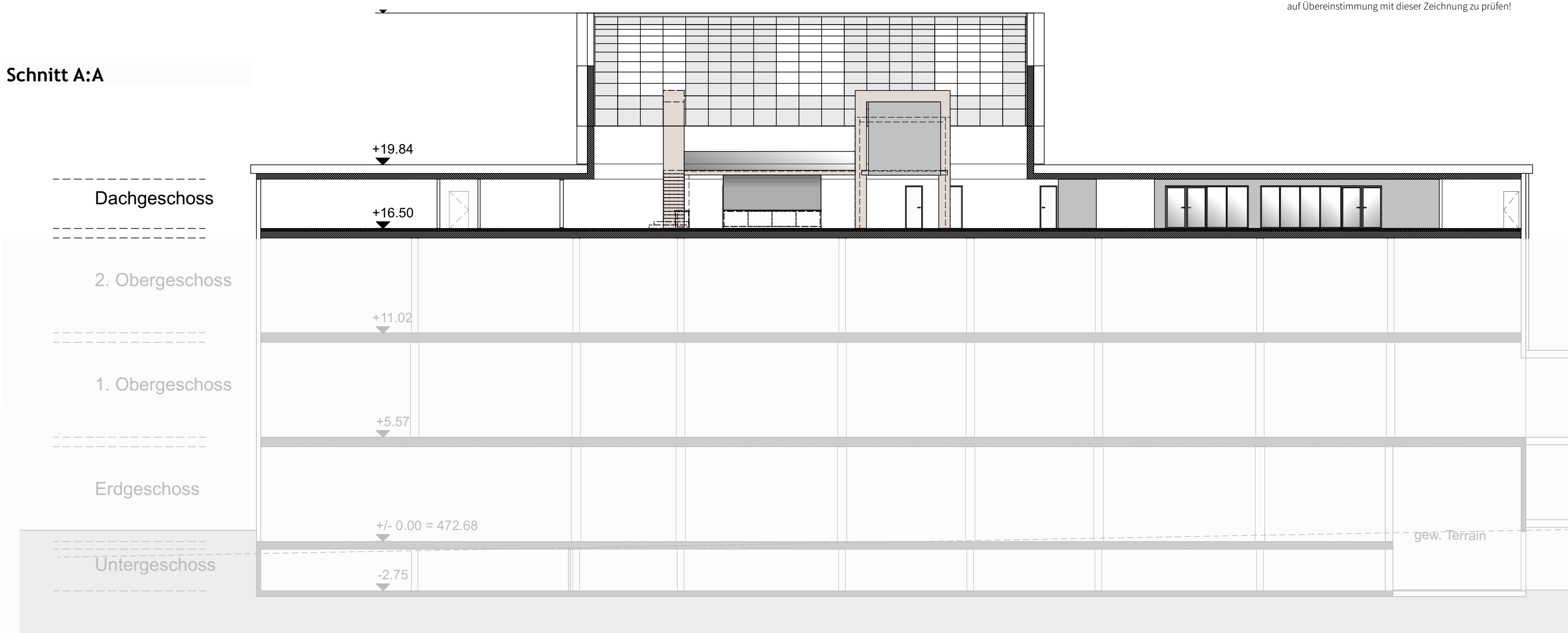
Schnitt D:D
