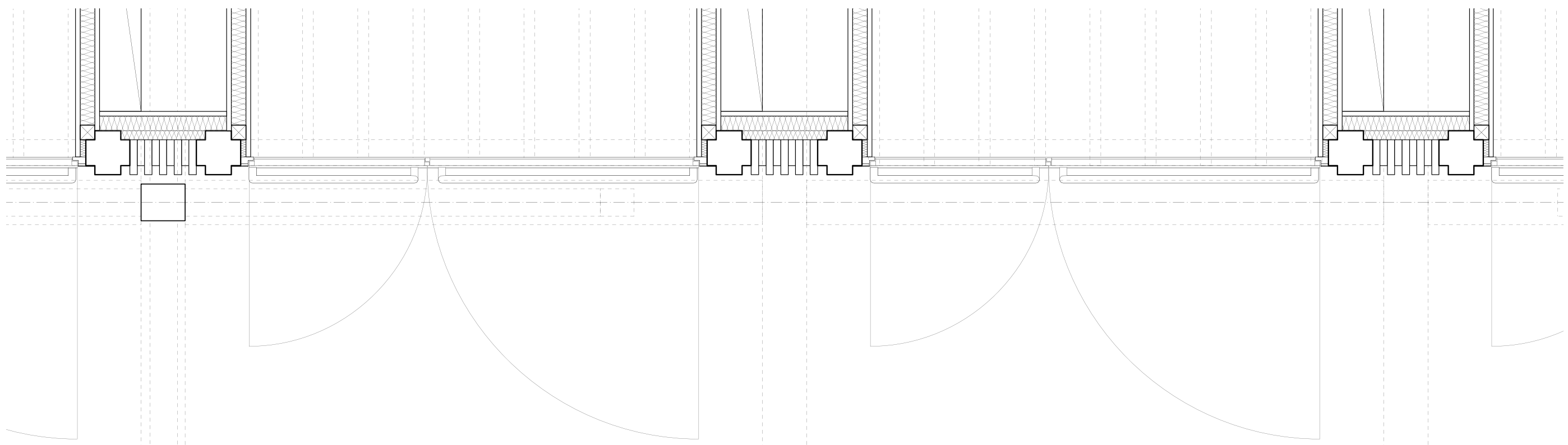
Grundriss Längswand Dachraum
