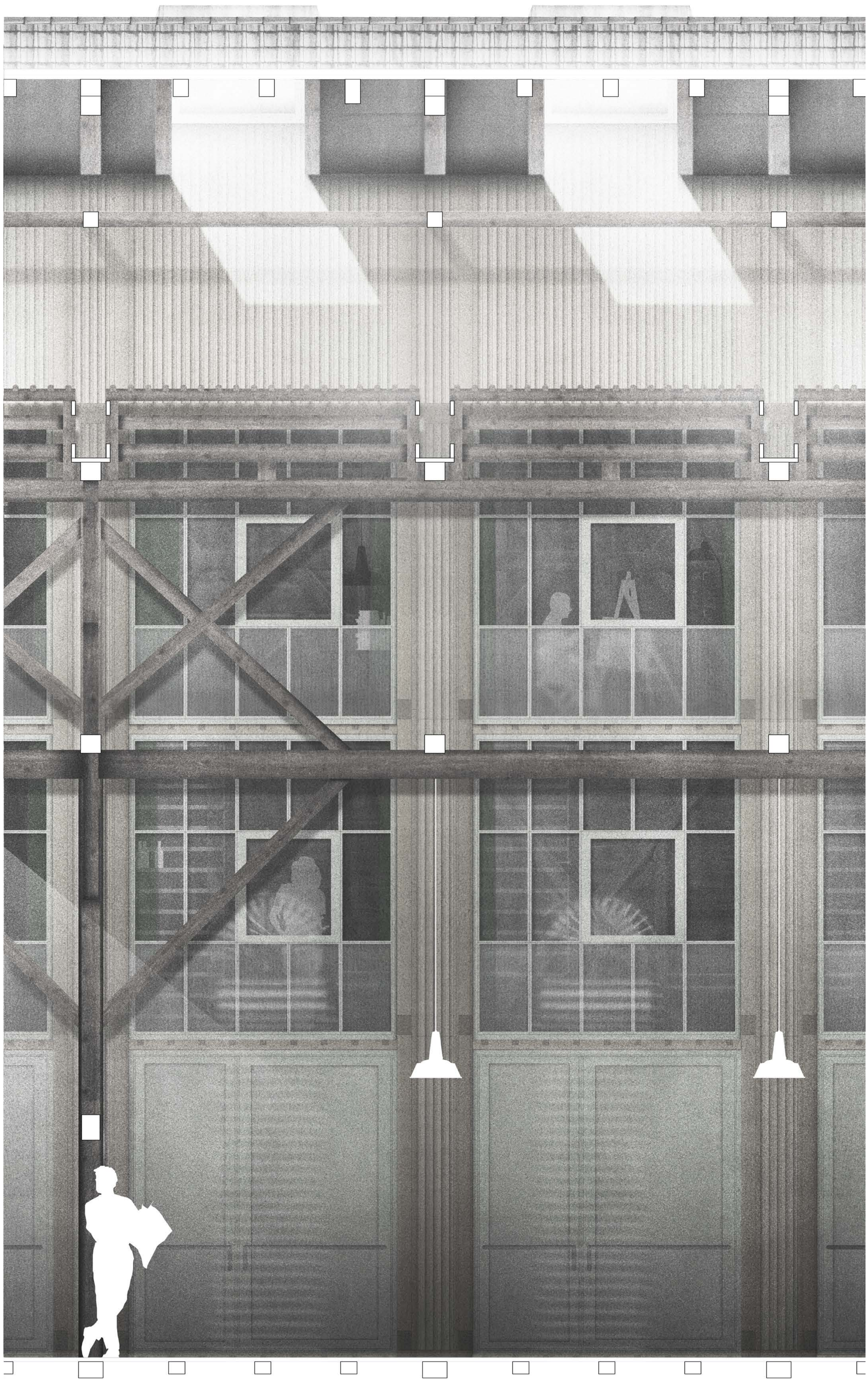
Ansicht Längswand Dachraum
