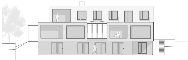
Ansicht Süd
