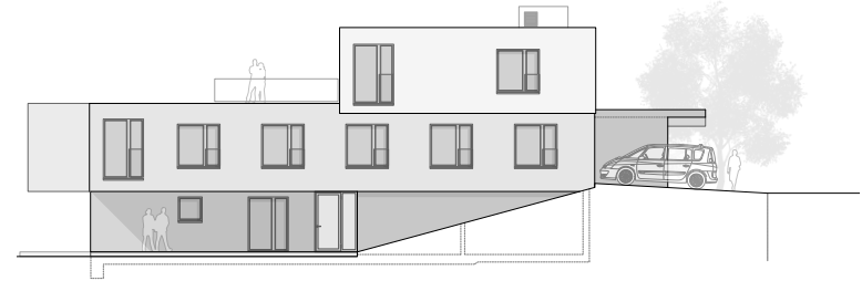
Ansicht Ost
