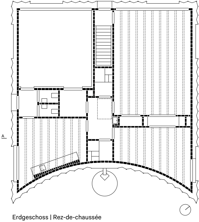
Erdgeschoss | Rez-de-chaussée
