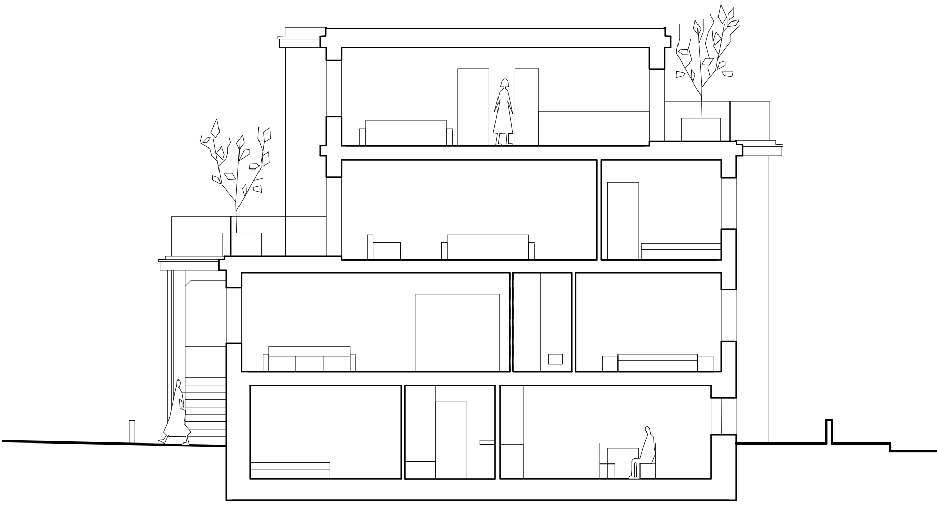
coupe AA
