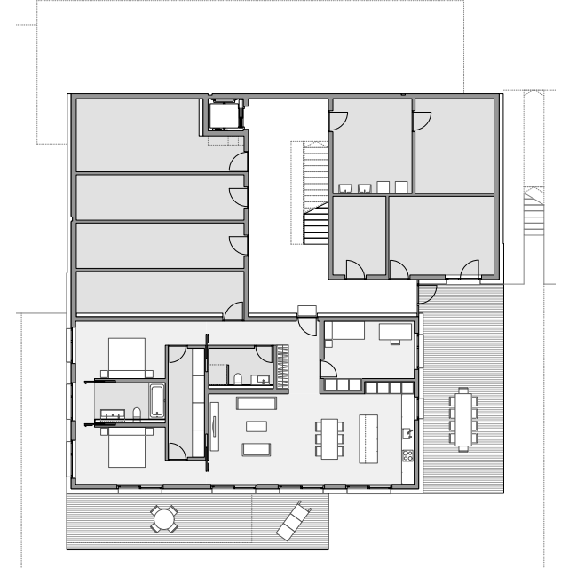
Gartengeschoss
