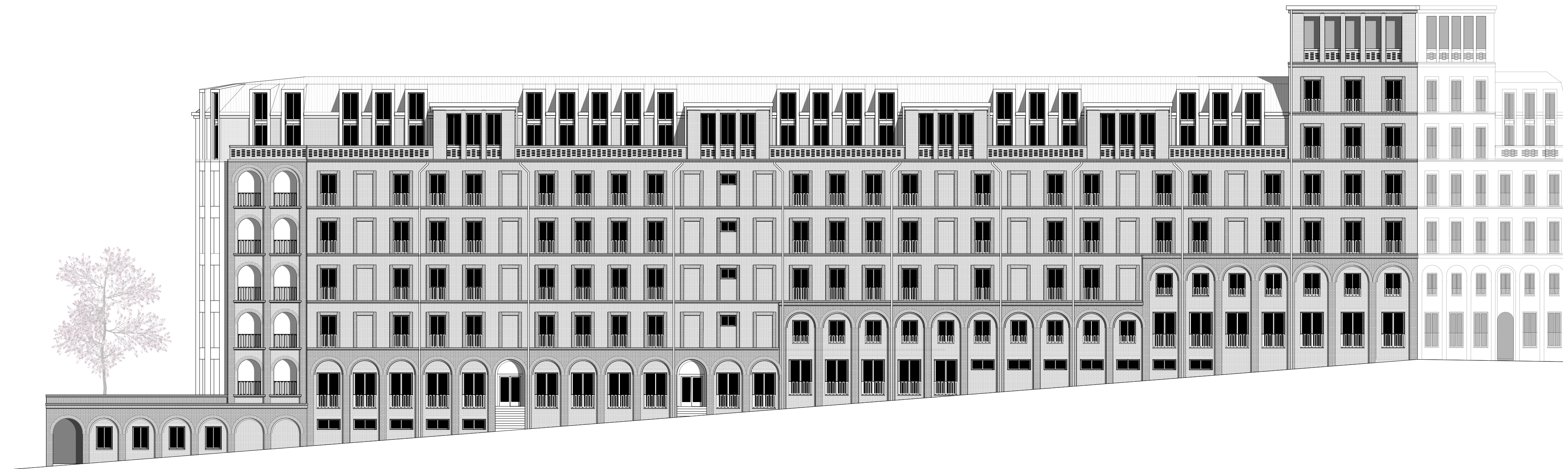
Südfassade, Bahngleis 1:200
