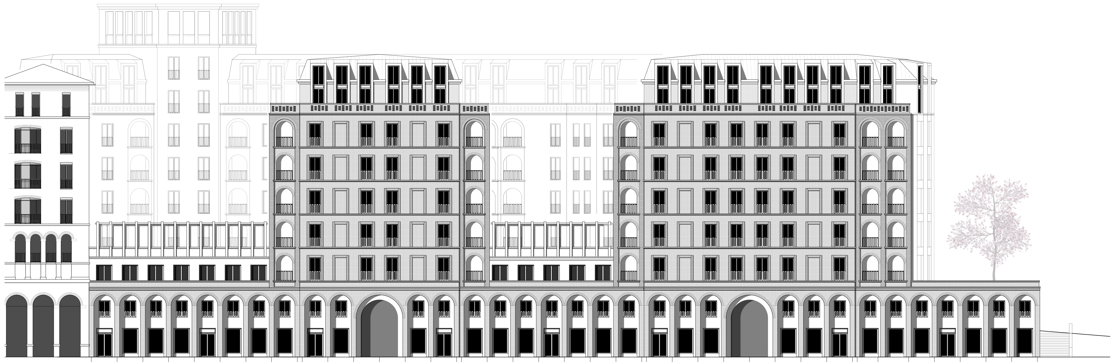
Südfassade, Bahngleis 1:200
