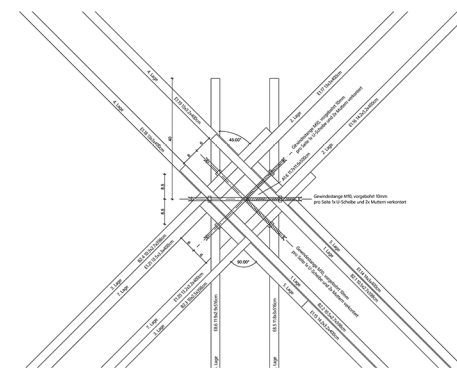
Grundriss Boden 1:10
