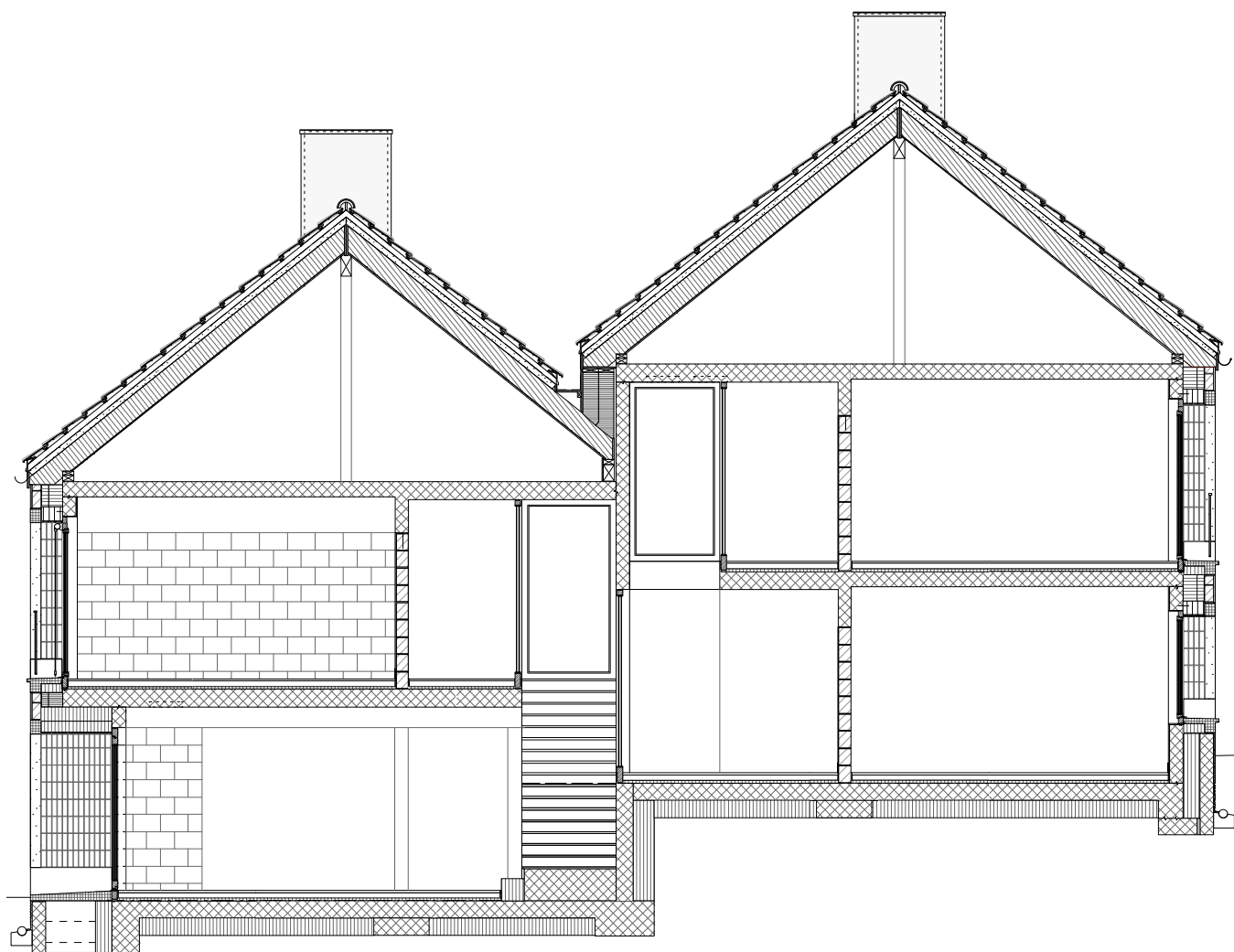
Coupe constructive 1:100
