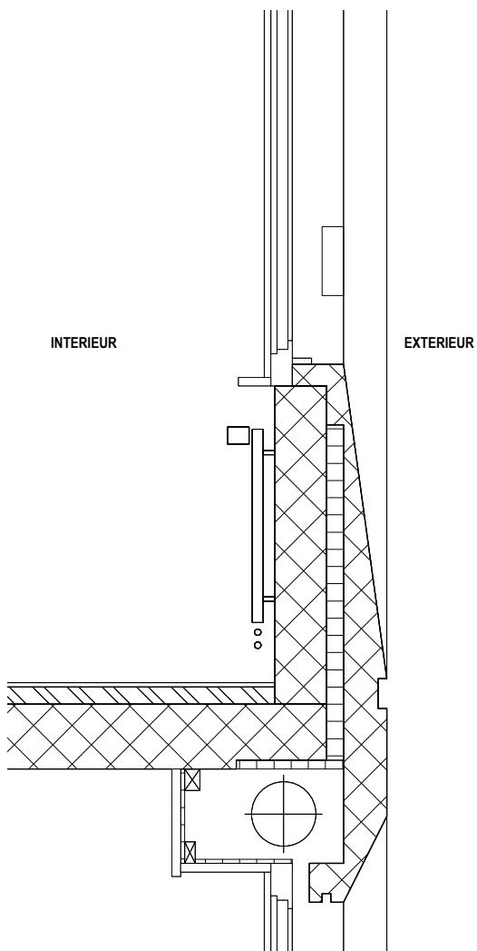
Coupe détail façade avant réhabilitation
