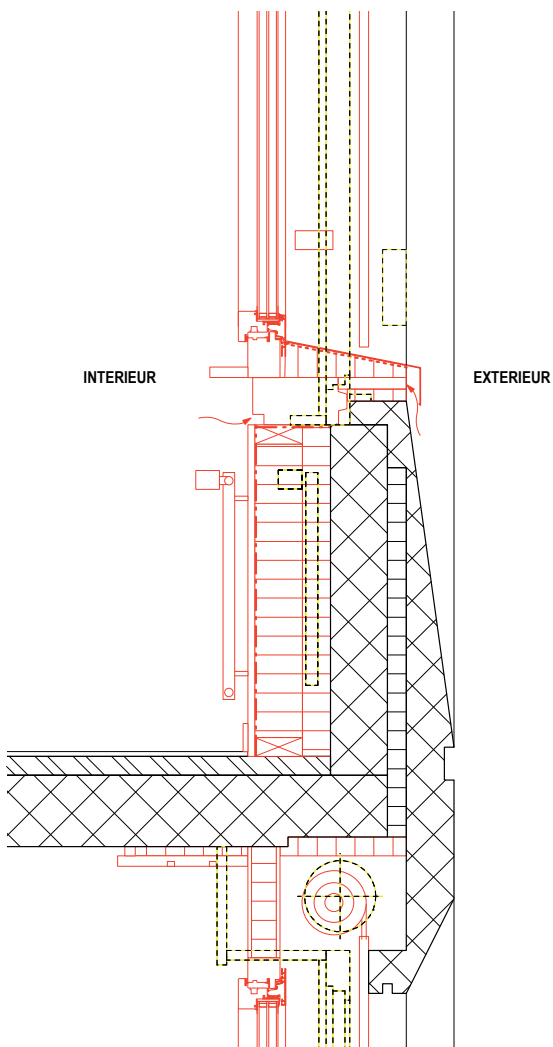
Coupe détail façade après réhabilitation
