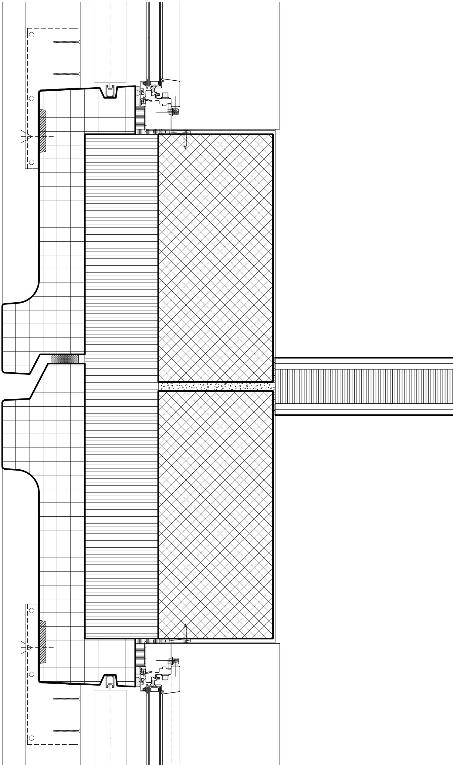
Schnitt 1:5
