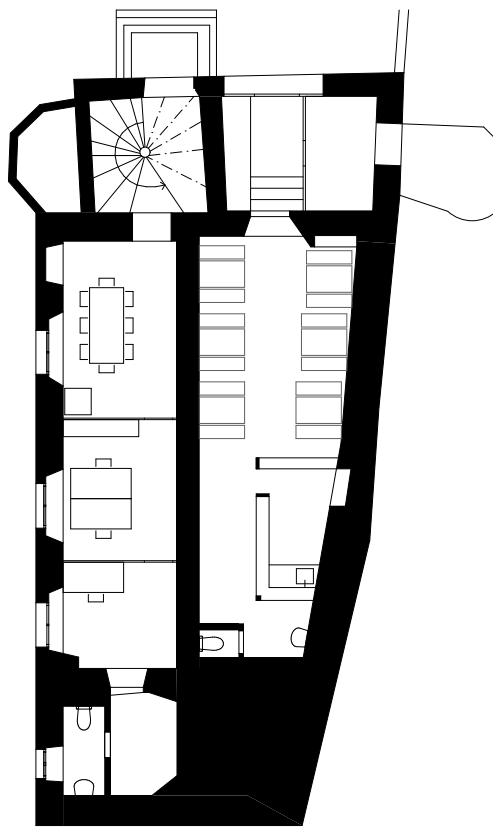
1.OG 1:200 0 1 2 5
