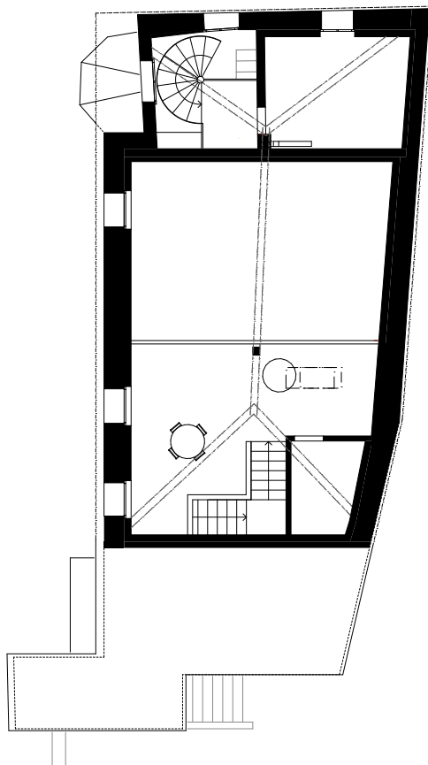
DG 1:200 0 1 2 5
