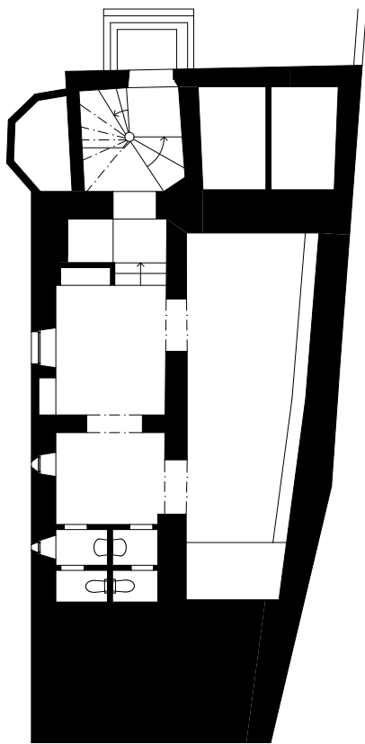
EG 1:200 0 1 2 5
