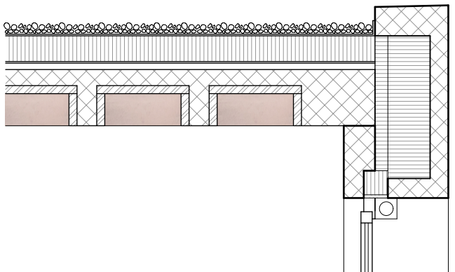
Dachdetail 1:33
