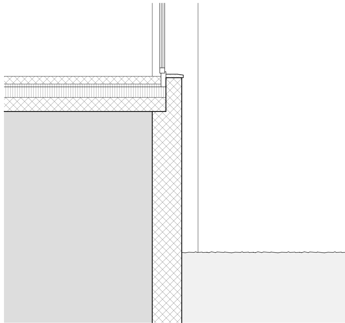
Sockeldetail 1:33
