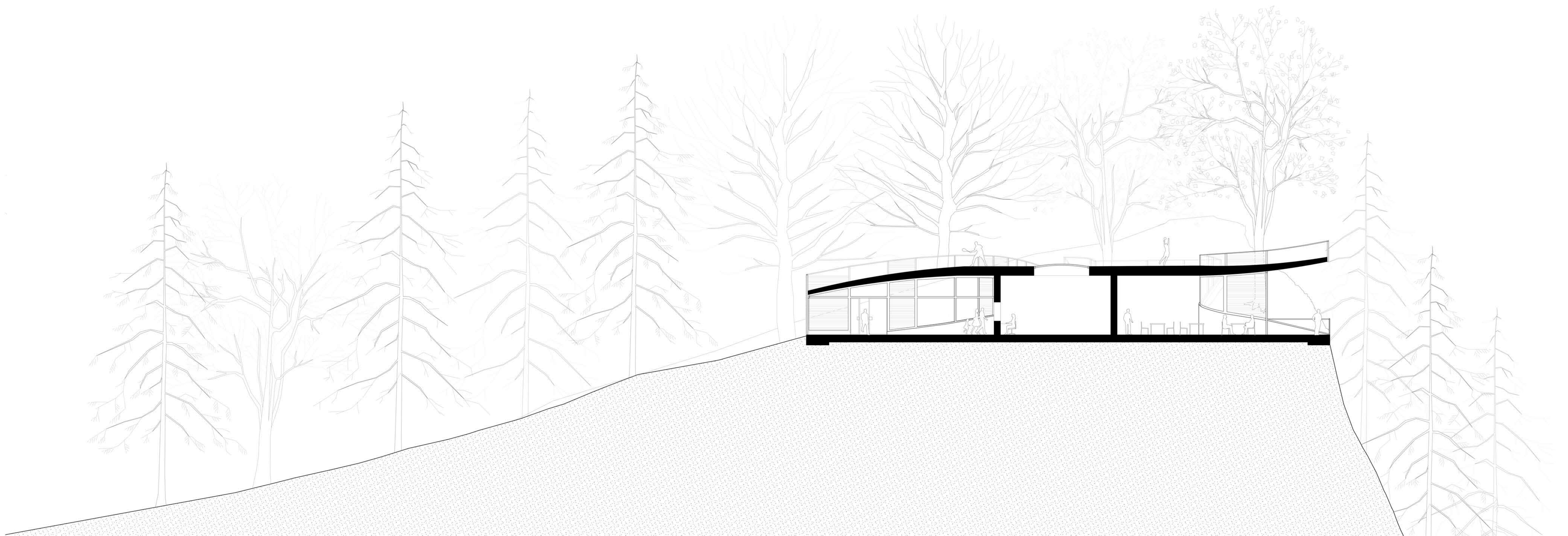
SECTION A-A, 1:100
