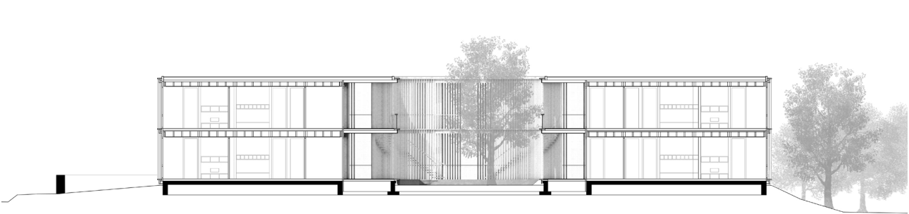
Längsschnitt | Coupe longitudinale
