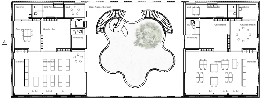
Obergeschoss | Étage
