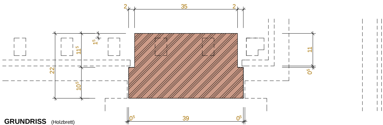
GRUNDRISS (Holzbrett)
