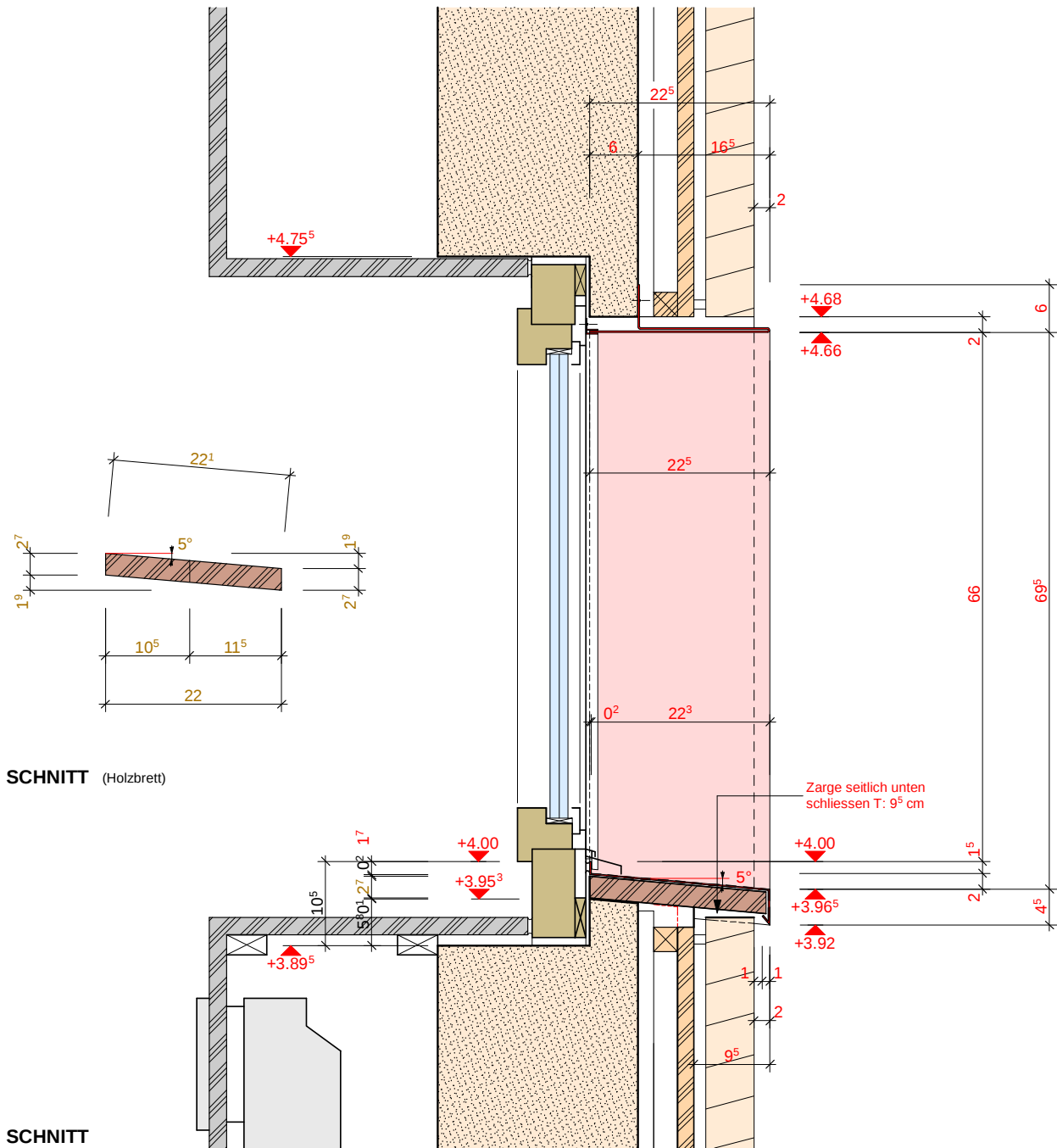
SCHNITT
