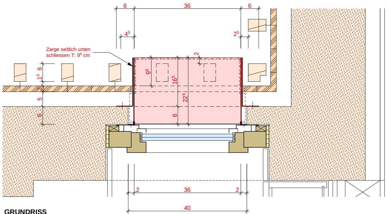
GRUNDRISS
