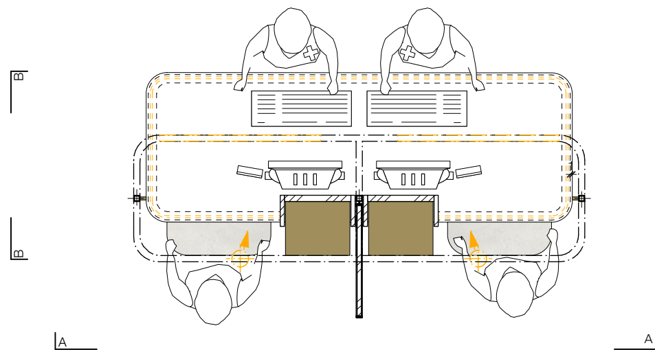
Grundriss
