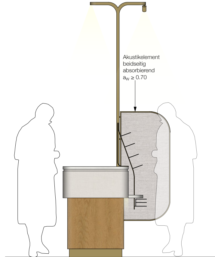
Ansicht B-B
