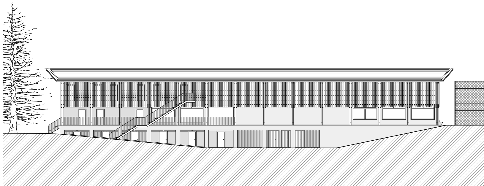
Ansicht Nord
