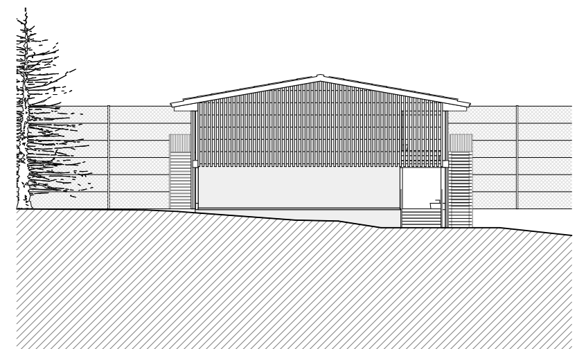
Ansicht Ost
