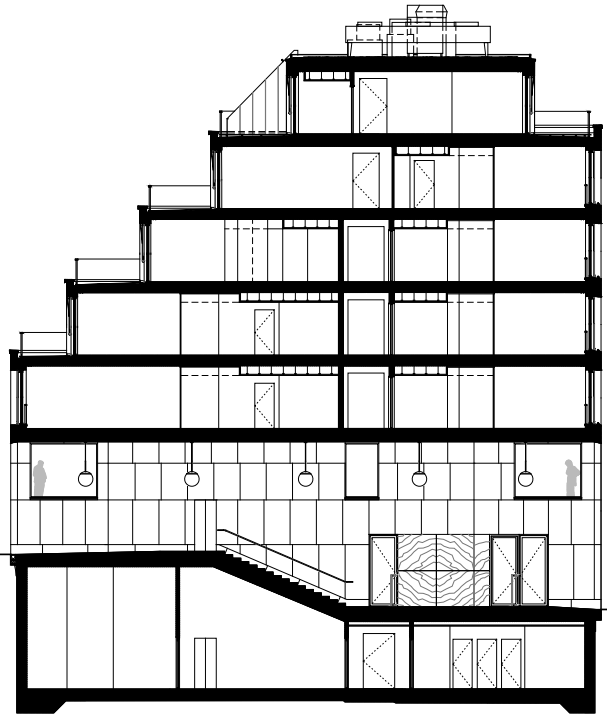
Schnitt | Coupe
