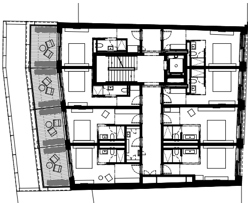
4. Obergeschoss | 4ème étage
