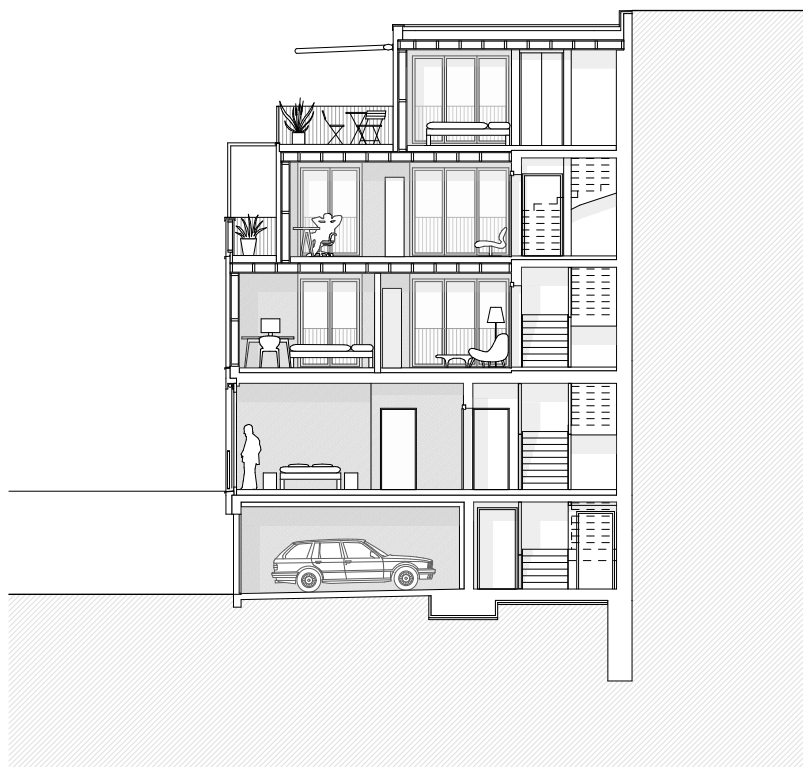
Querschnitt
