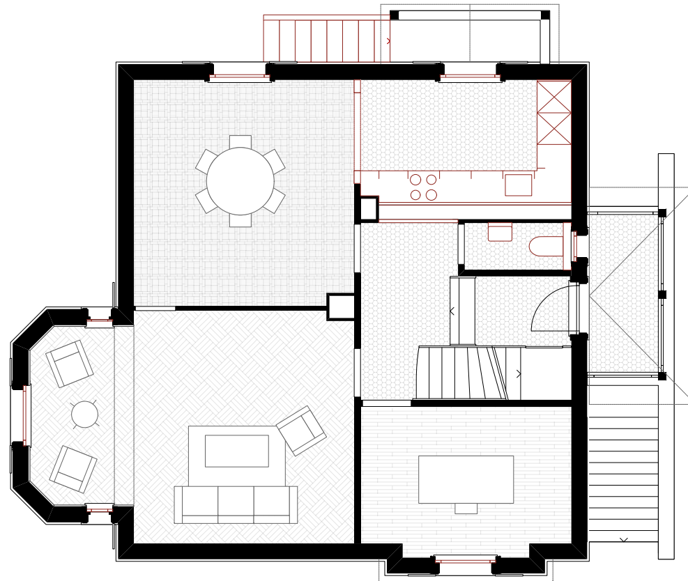
Erdgeschoss 1:100
