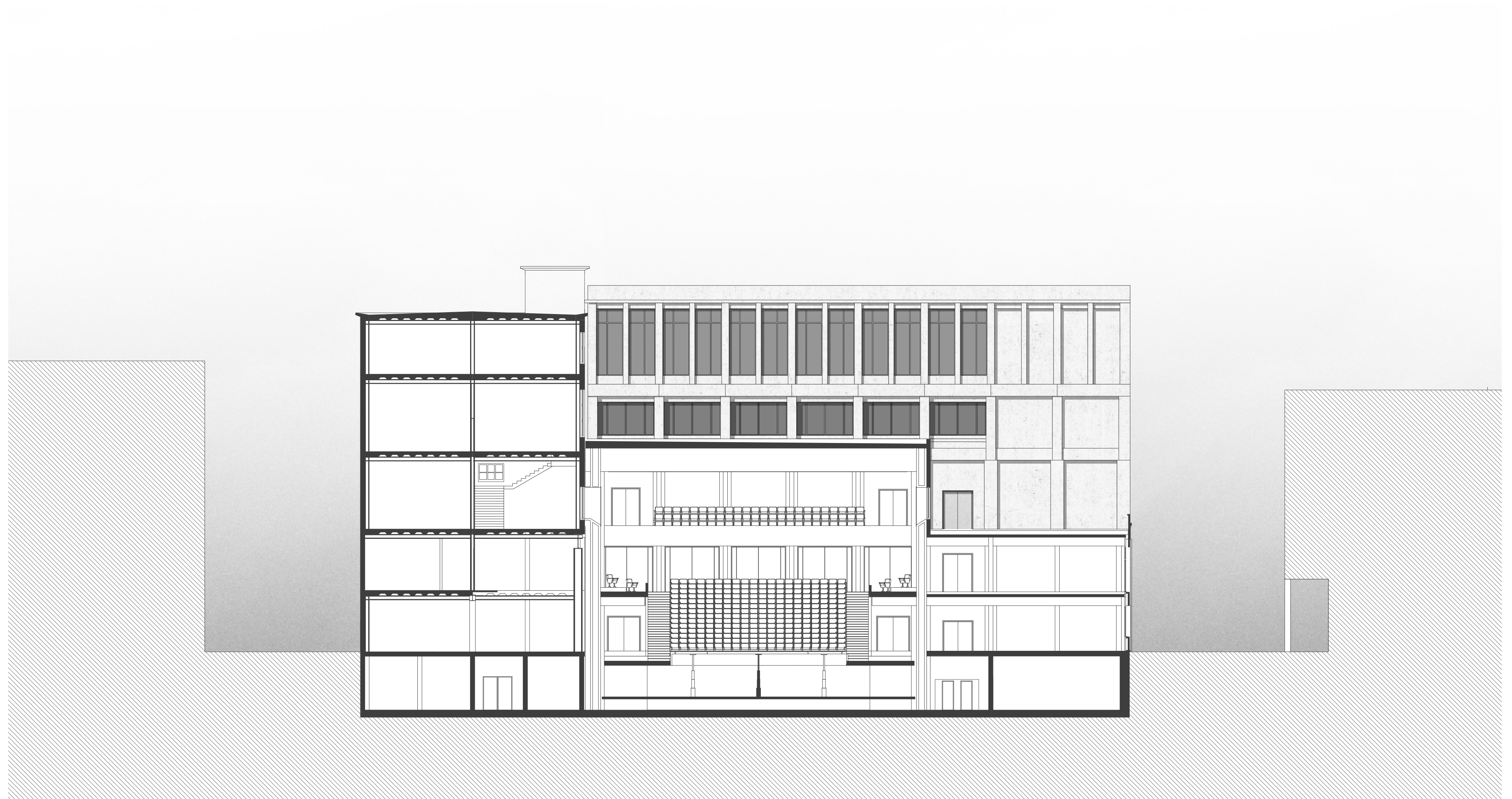
Querschnitt Halle | 1:200
