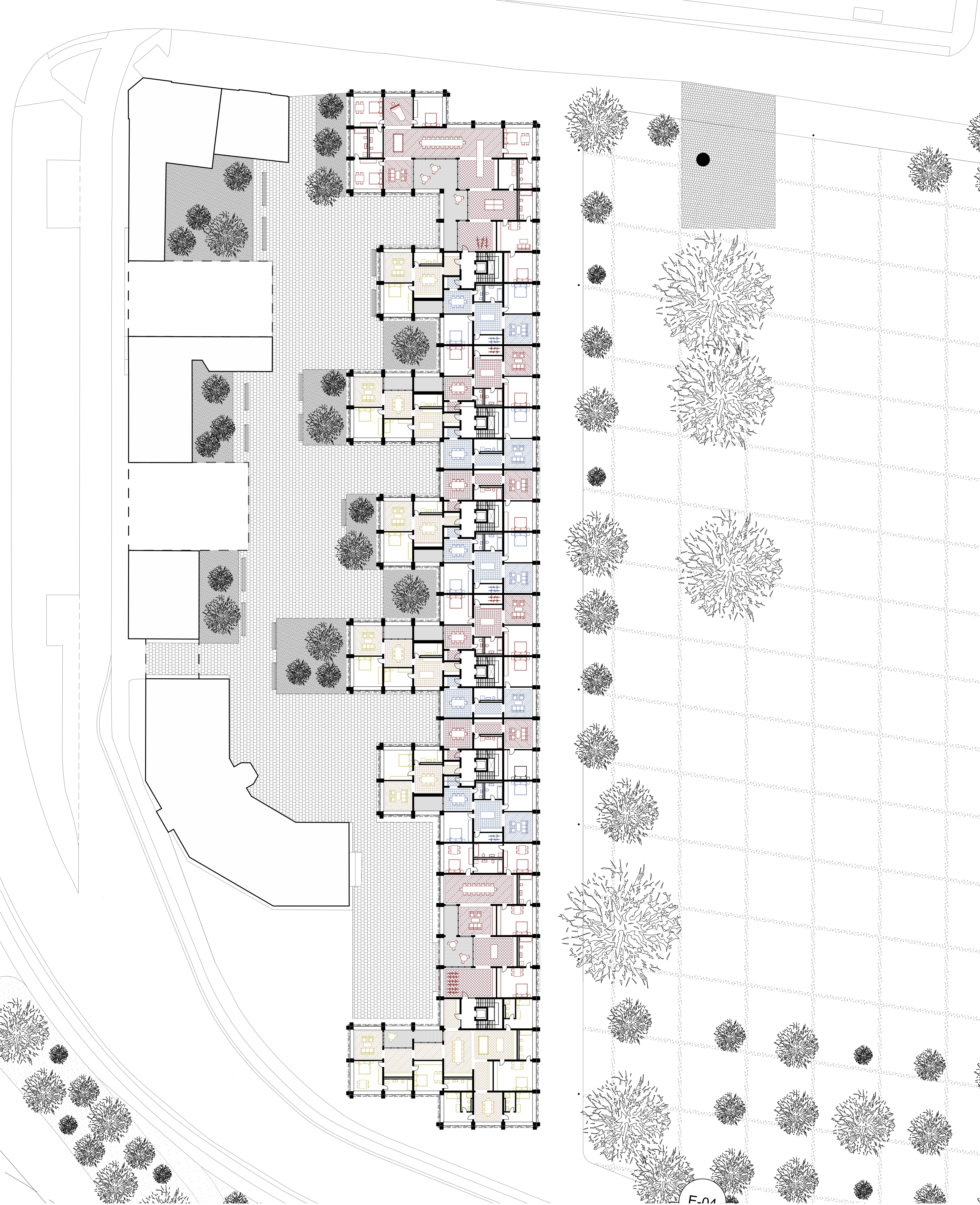
Etage type 1/350
