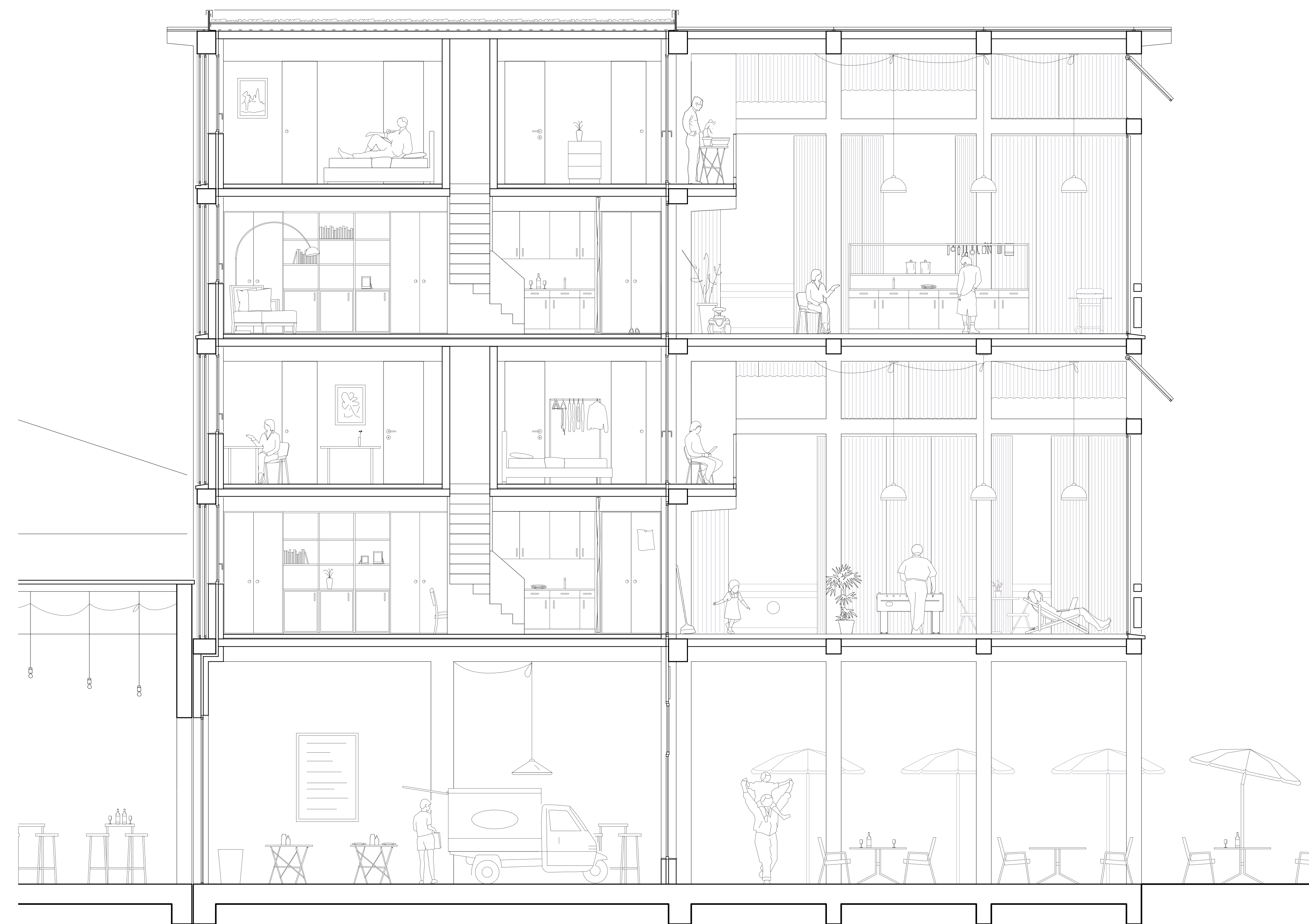
Detailanschnitt Haus 1 1:50
