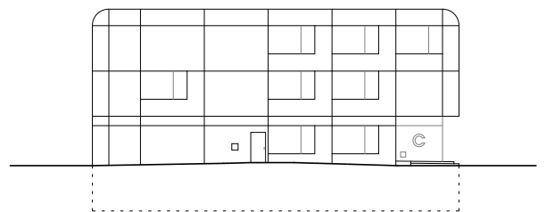
façade sud
