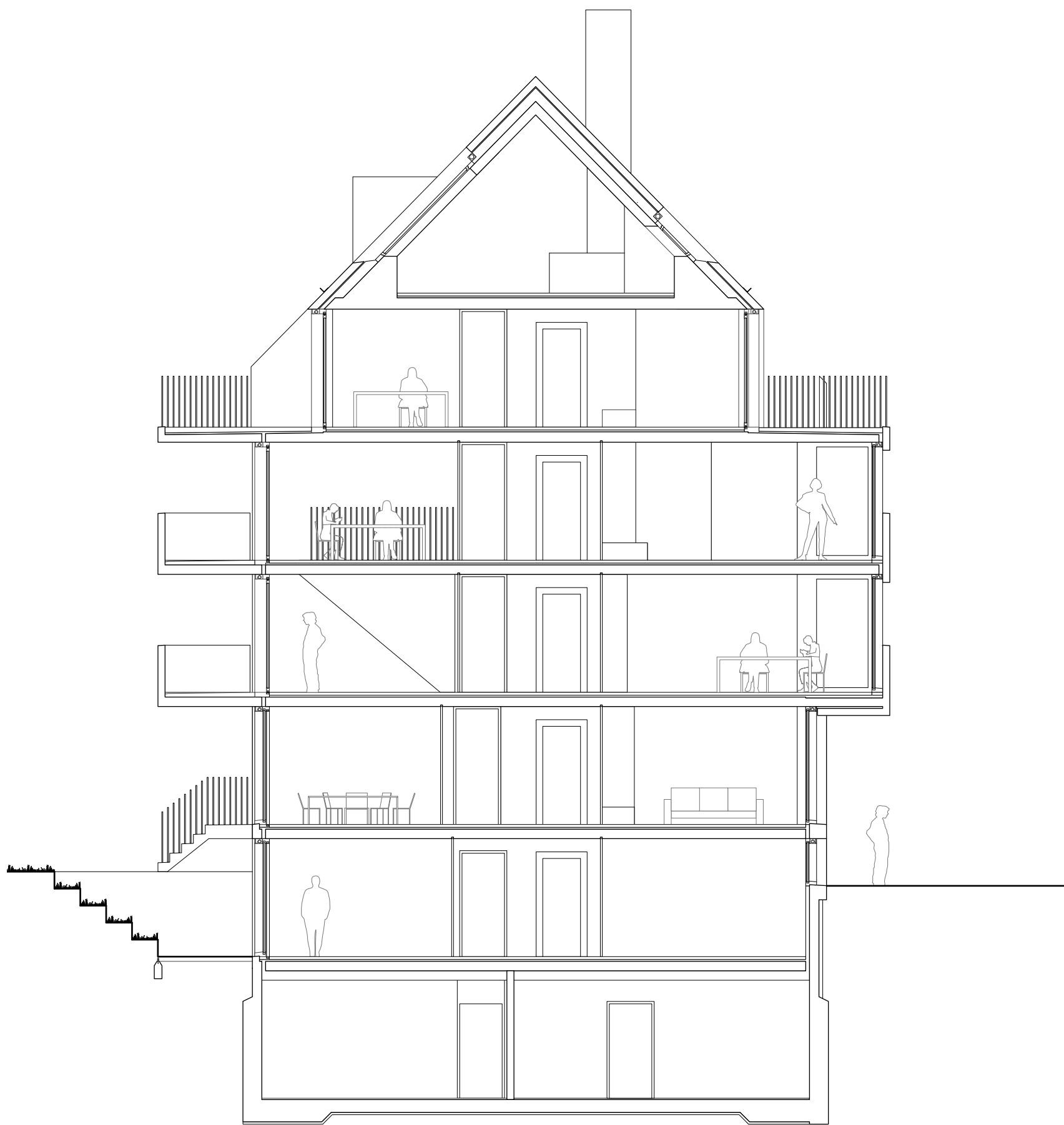
Längsschnitt I 1:100
