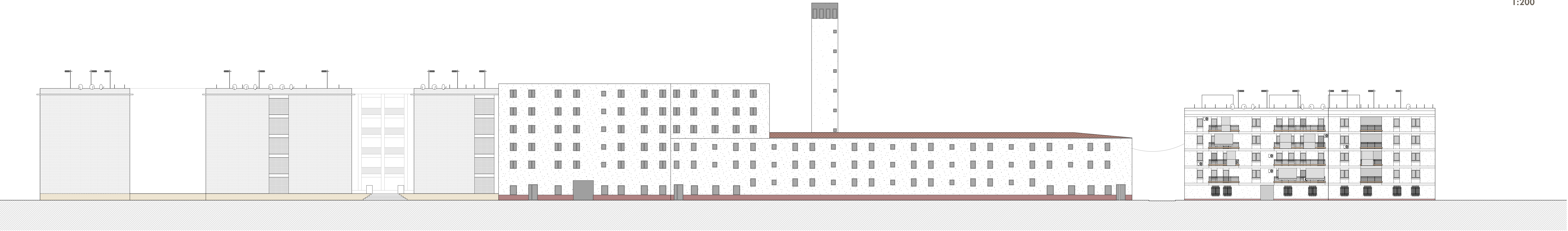
FACHADA NORTE 1:200
