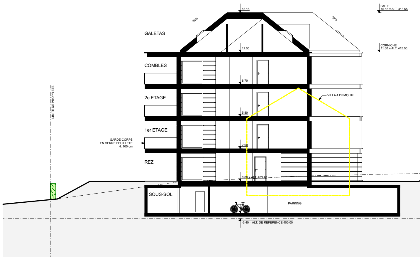
COUPE B-B
