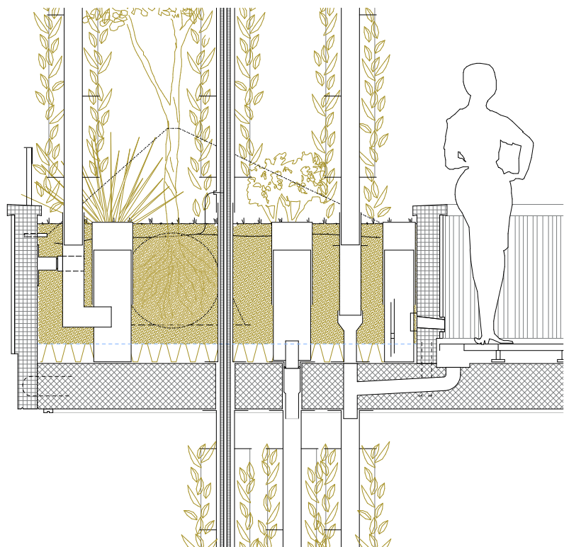
Gartenhochhaus Aglaya Detailschnitt Pflanztrog
