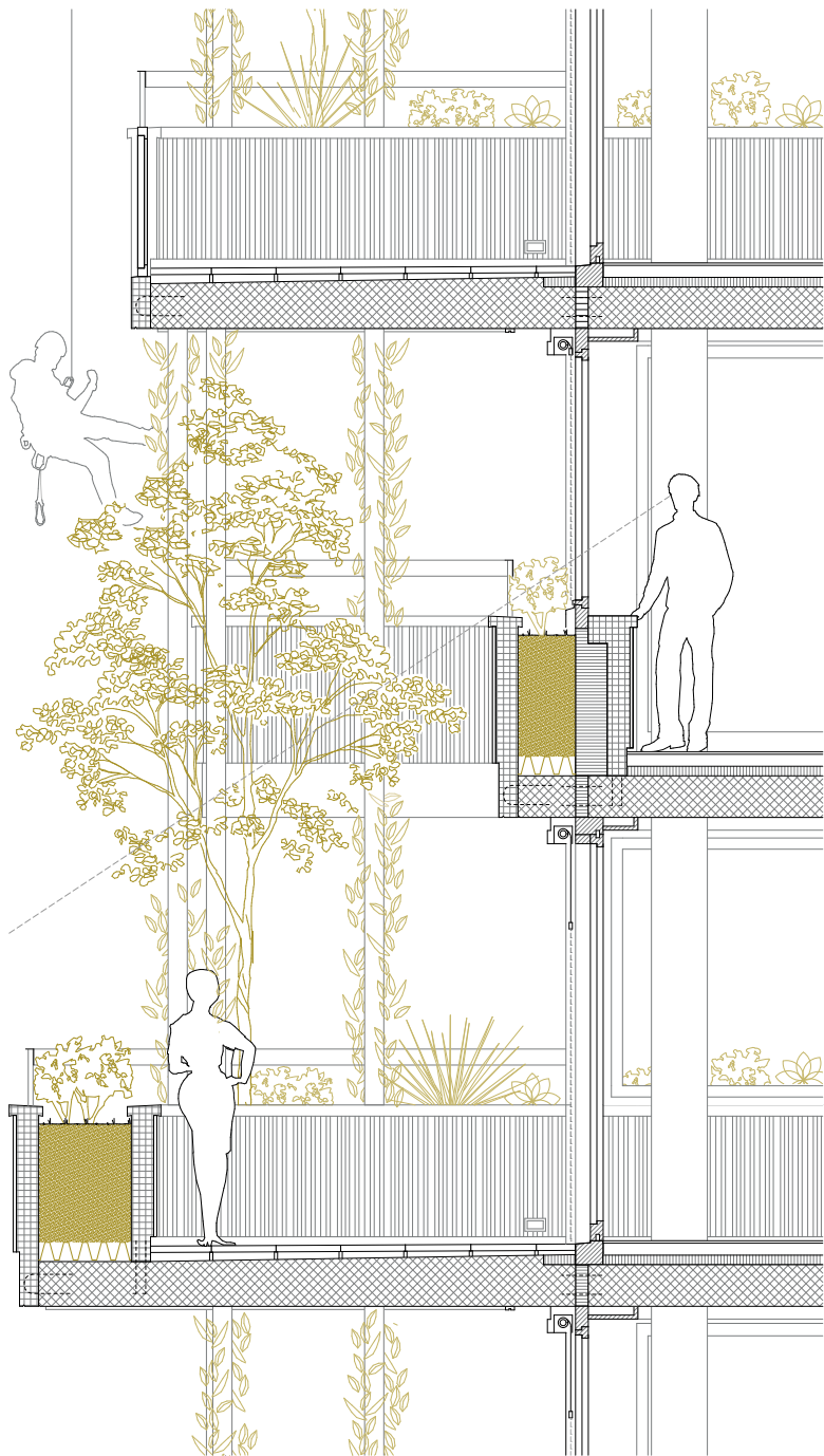
Gartenhochhaus Aglaya Detailschnitt Balkon
